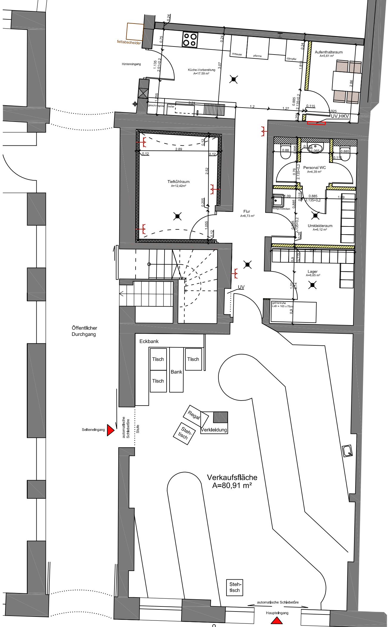
Stadtplatz 5, Vilsbiburg - Erdgeschoß Gewerbefläche A=144,42m 2
