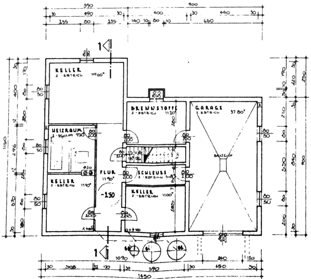
KELLER
