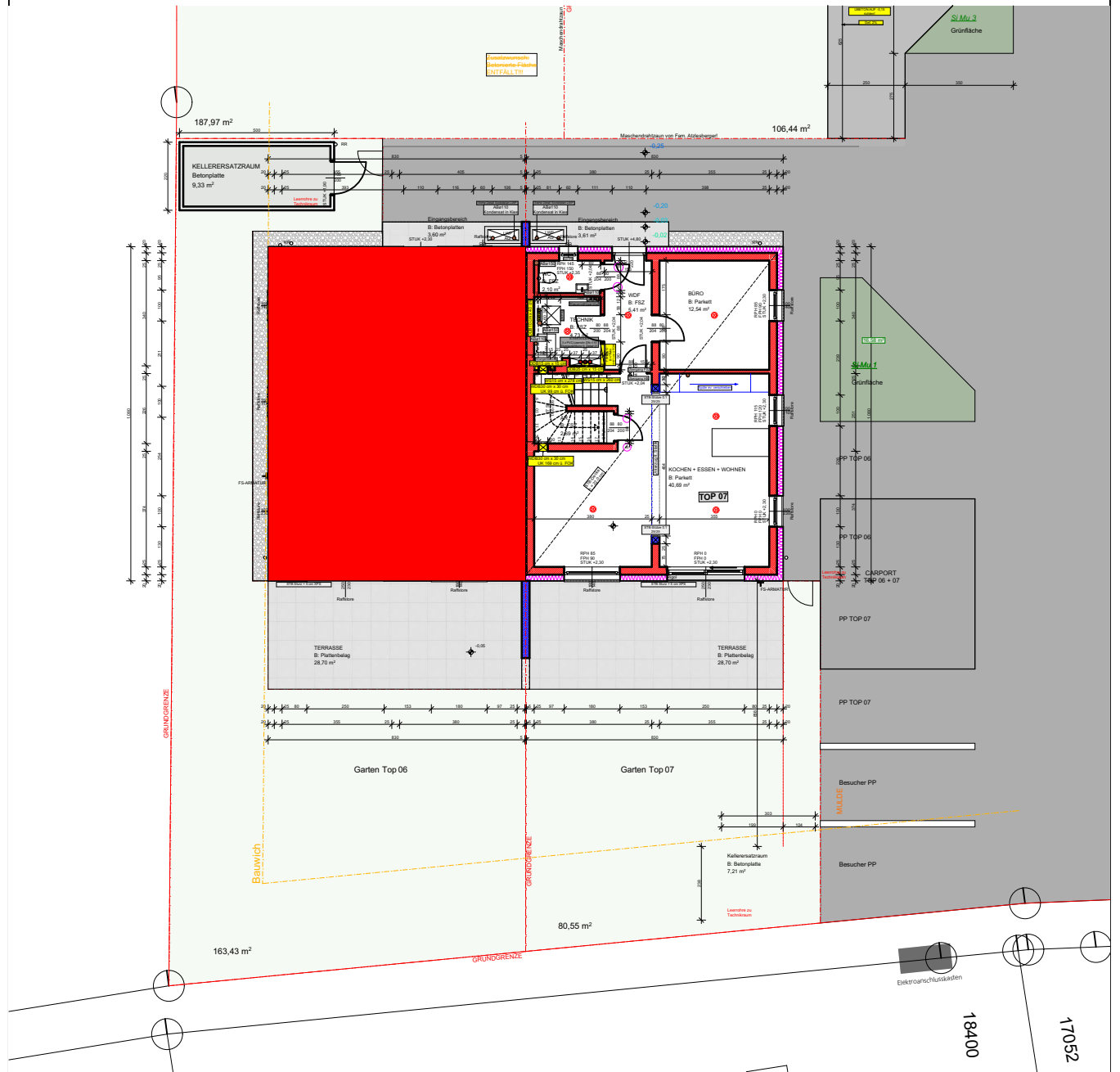
Übersichtsplan - M 1:200
