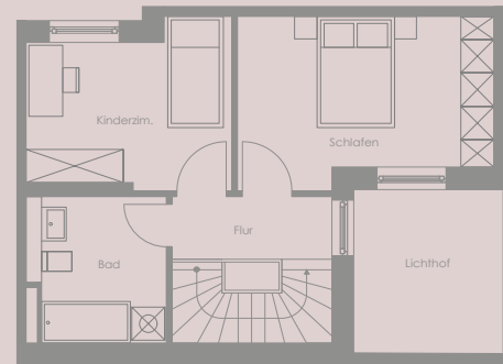
2. OBERGESCHOSS
