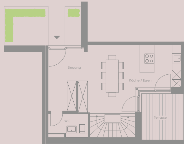
ERDGESCHOSS
