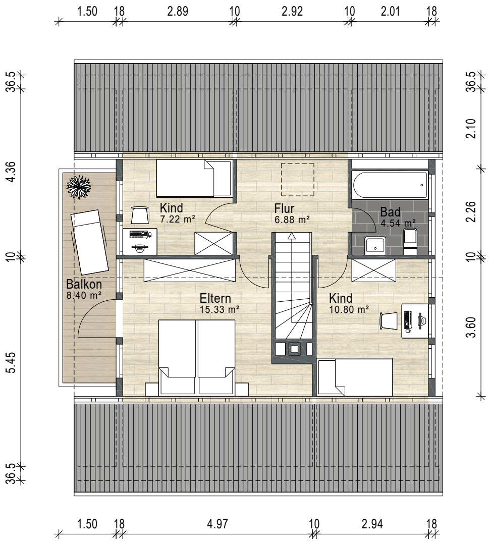
Dachgeschoss
