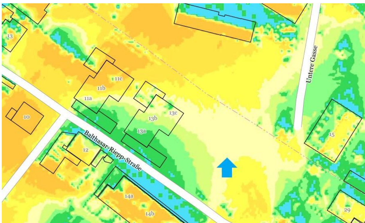
Sonnenscheindauer 21. Dez
