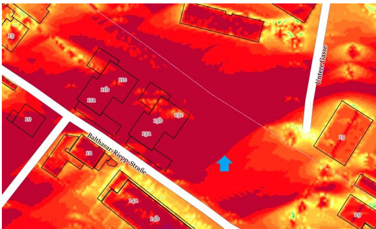
Sonnenscheindauer 21. Jun
