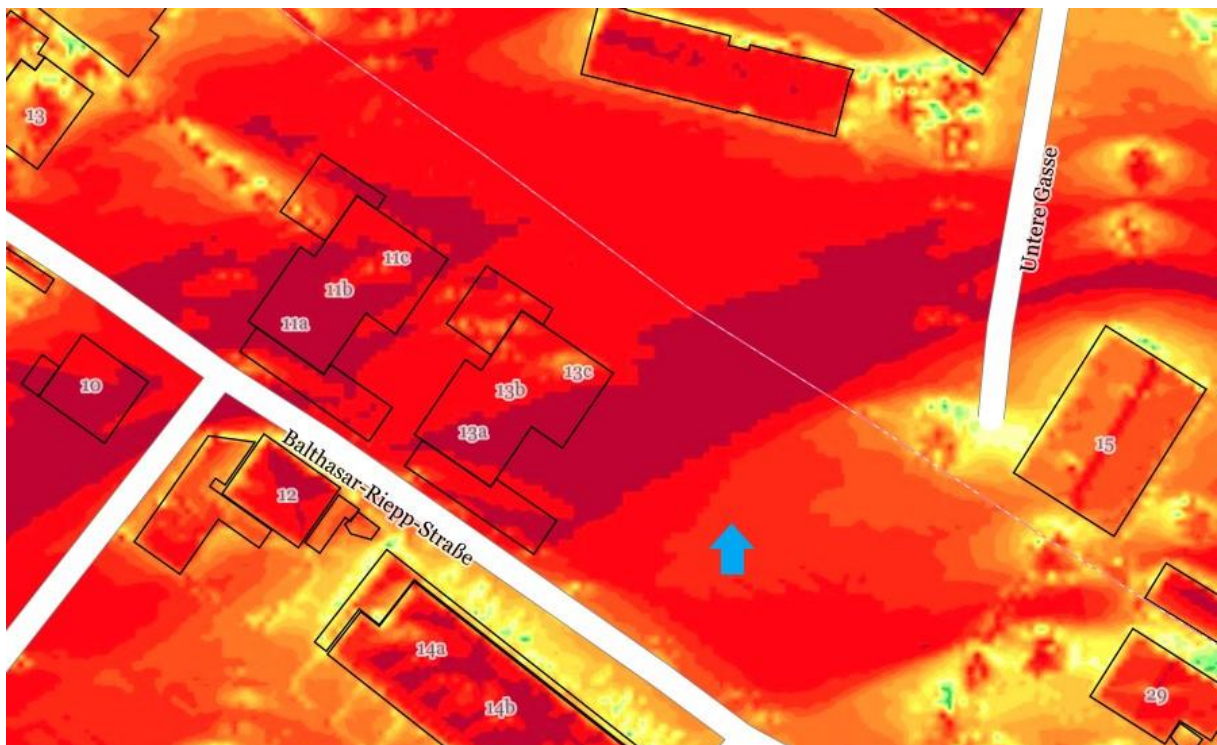
Sonnenscheindauer 21. Mai
