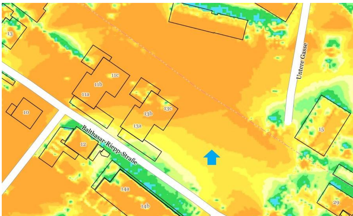
Sonnenscheindauer 21. Feb
