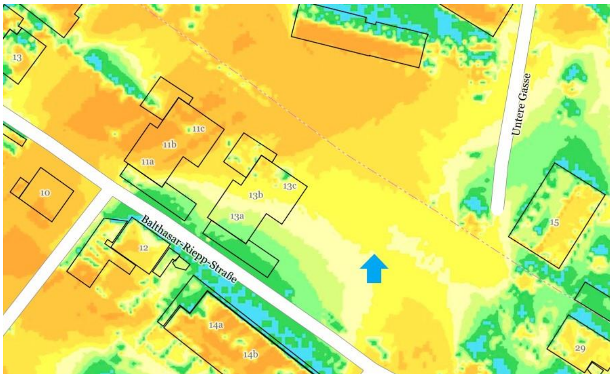
Sonnenscheindauer 21. Jan
