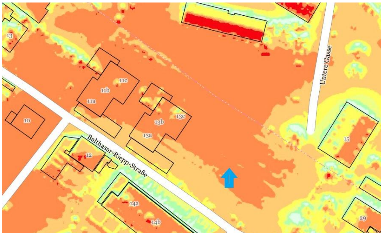
Solarstrahlung Jahr
