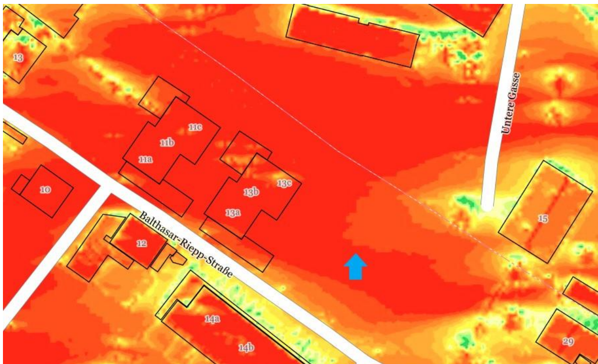
Sonnenscheindauer 21. Apr
