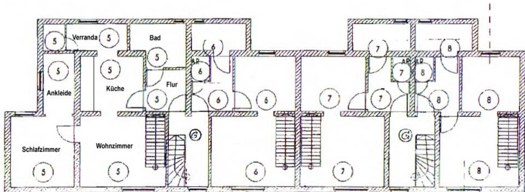
OBERGESCHOSS
