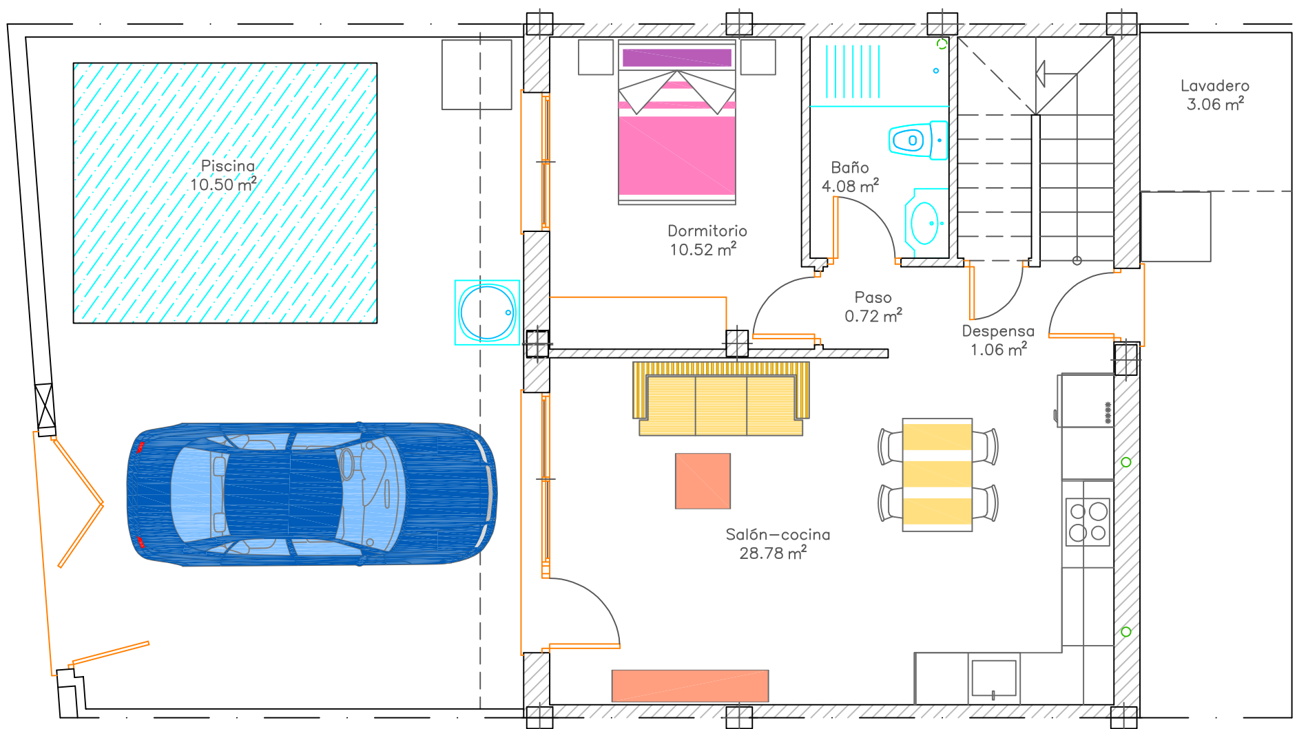
PLANTA 0, S.C.= 62.03M2
