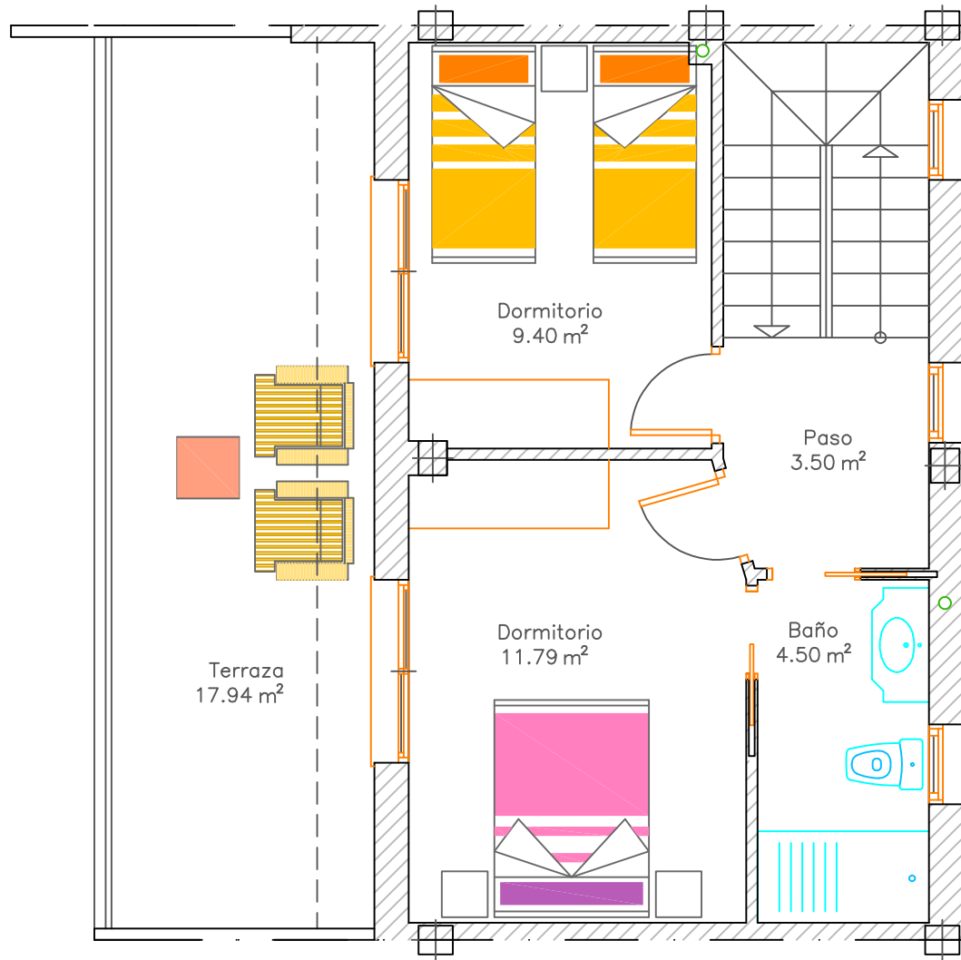
PLANTA 1, S.C.= 43.20 M2
