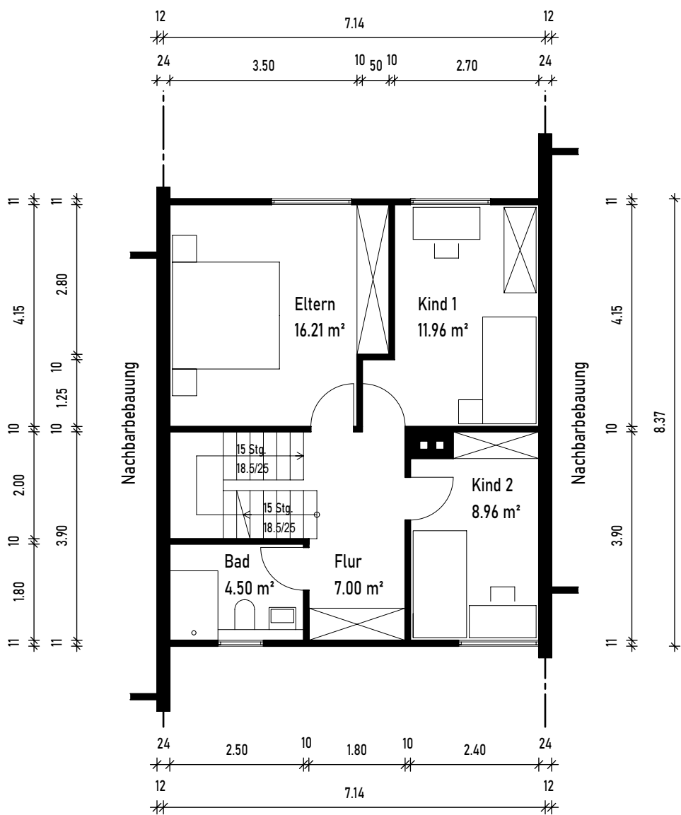
Obergeschoss
