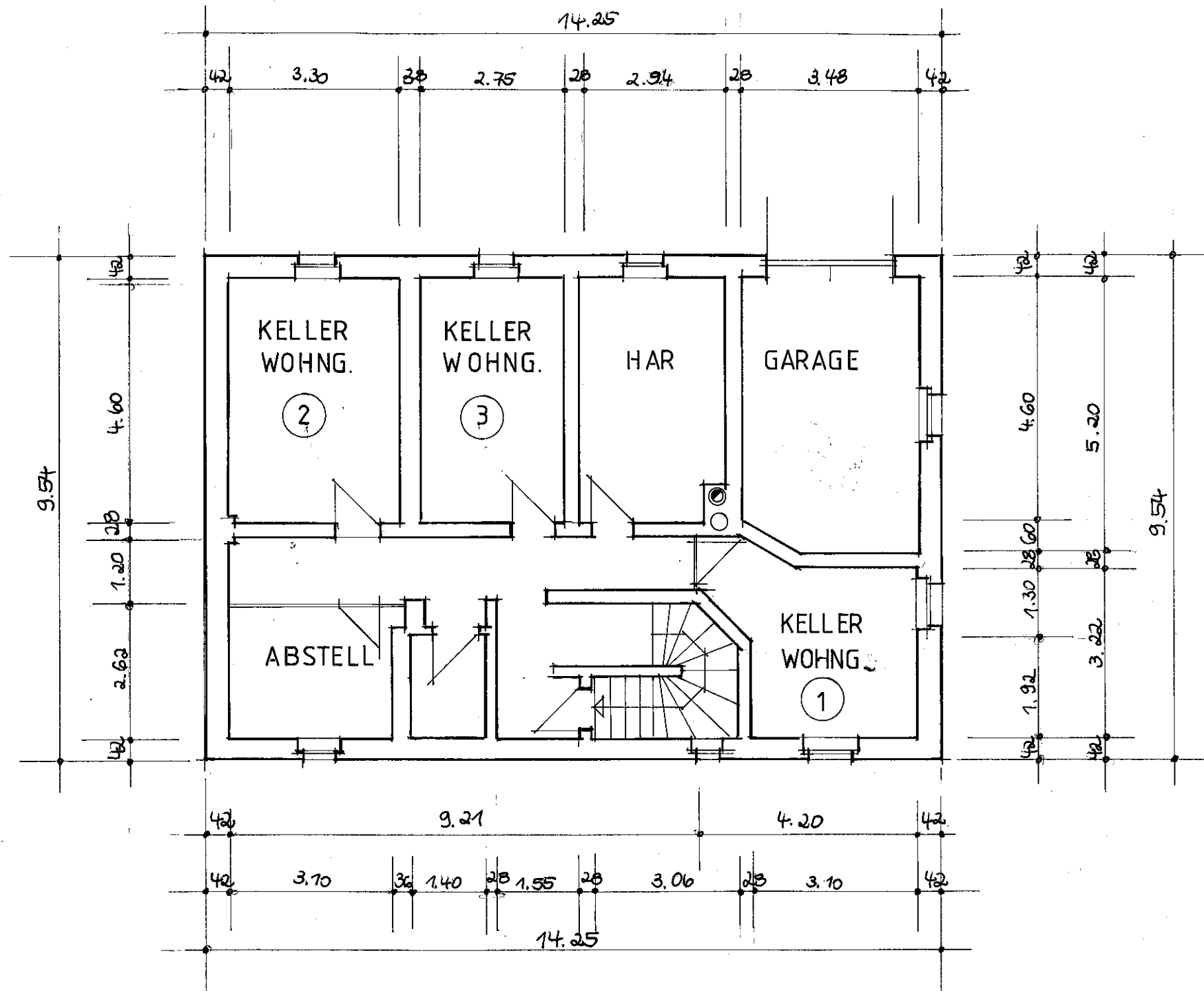
KELLERGESCHOSS M 1:100
