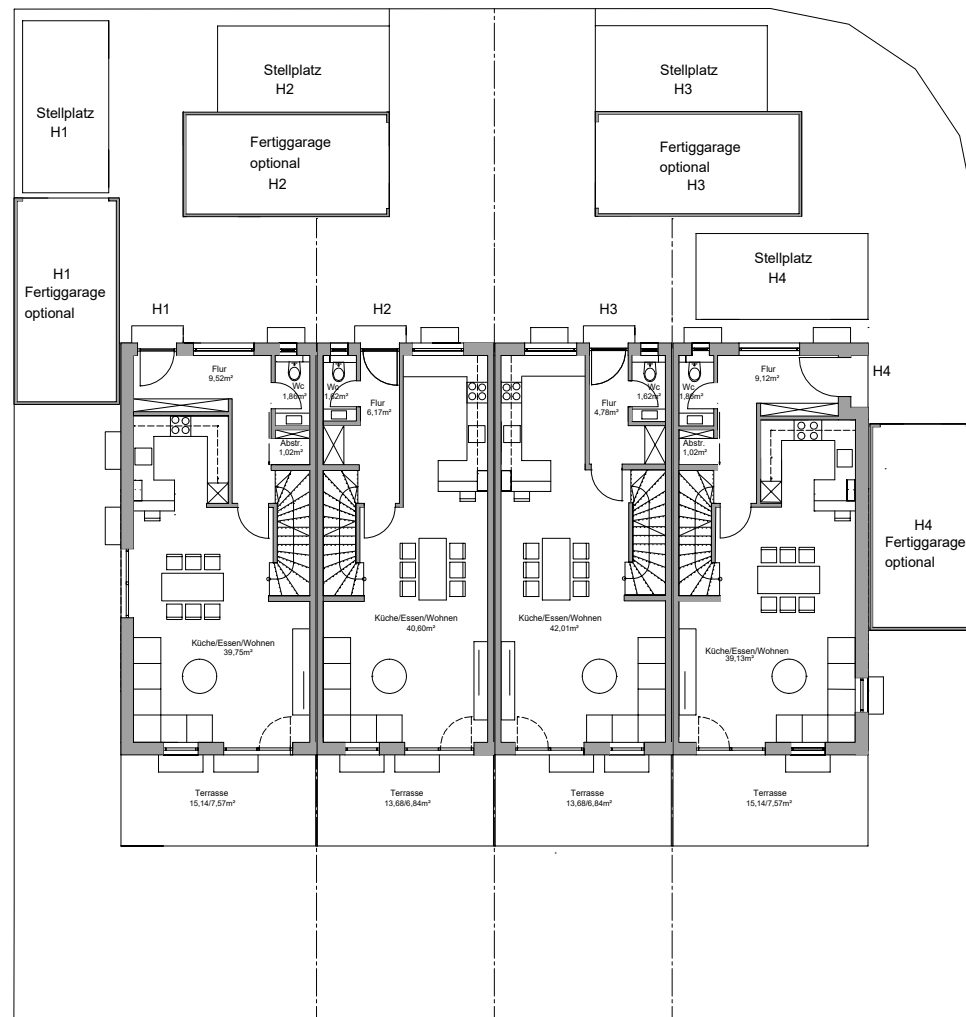
GRUNDRISS REIHENHAUS ERDGESCHOSS
