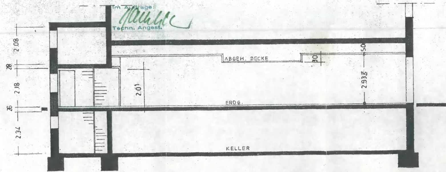
SCHNITT
