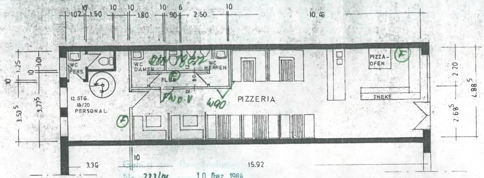
ERDGESCHOSS
