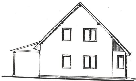
ANSICHT - NORD
