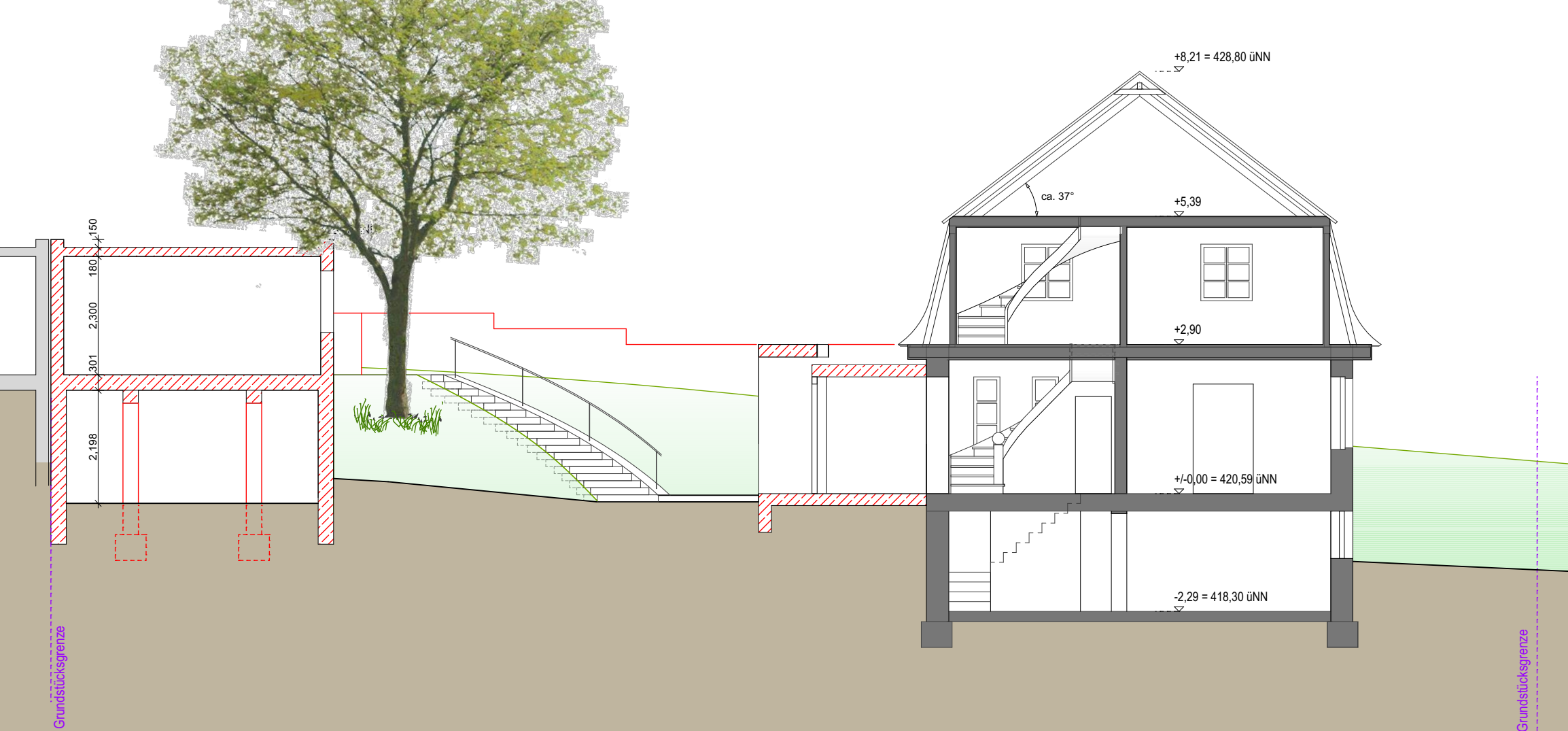
Schnitt A-A
