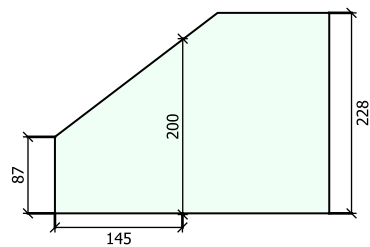
Ansicht Dachschräge
