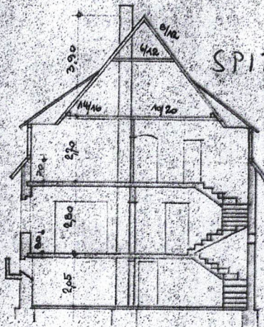
Schnitt
