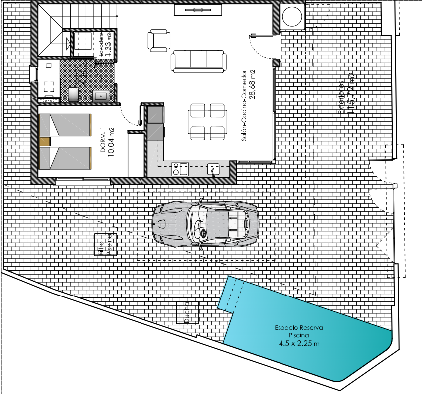
PLANTA BAJA
