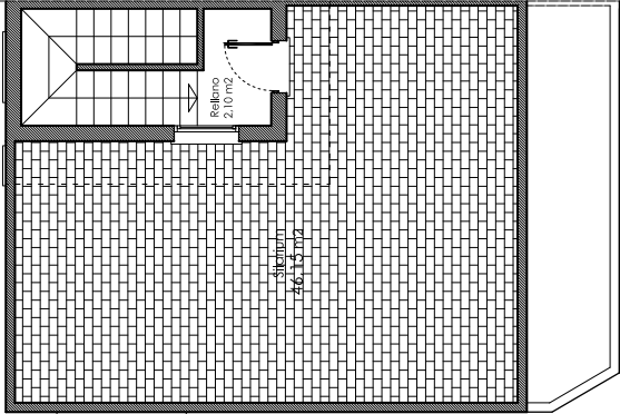
PLANTA SOLARIUM
