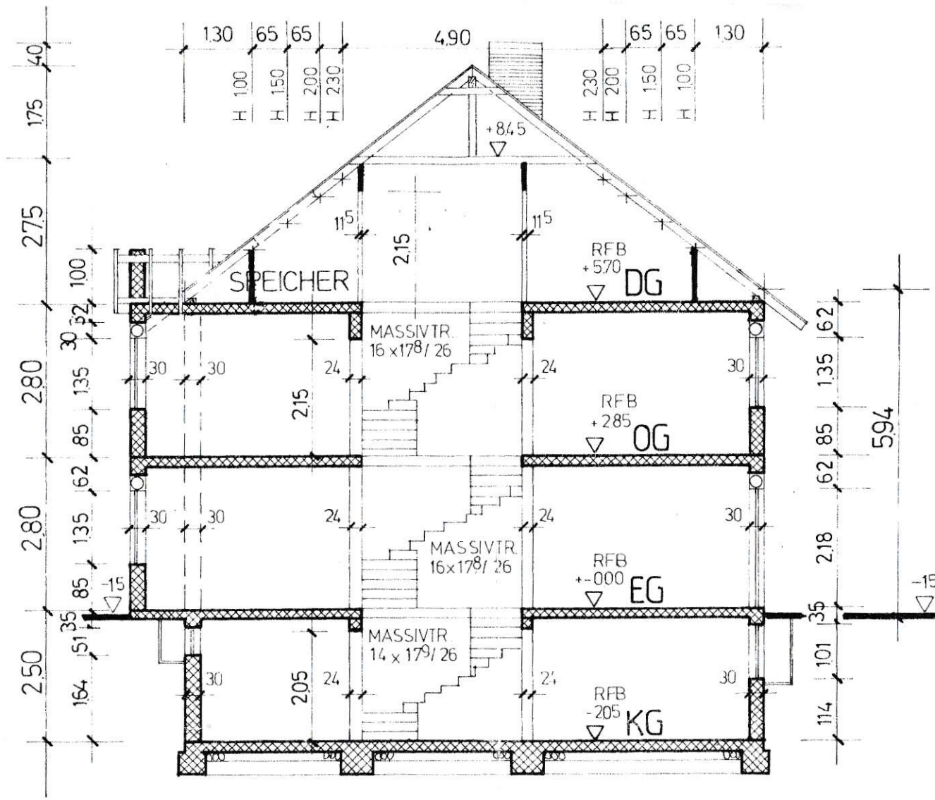
SCHNITT A - A WOHNHAUS 1
