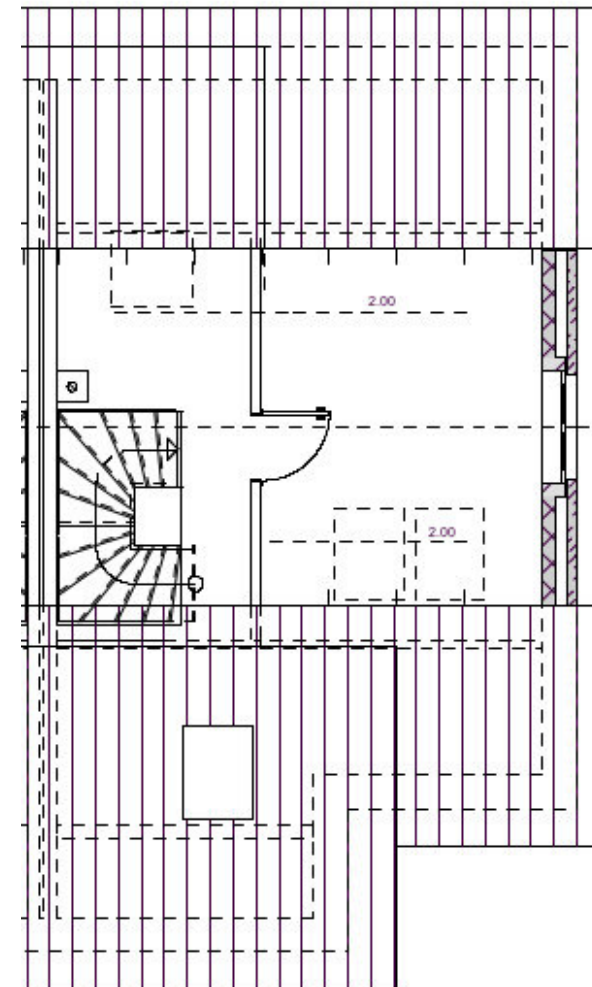
Grundriss Galeriegeschoss
