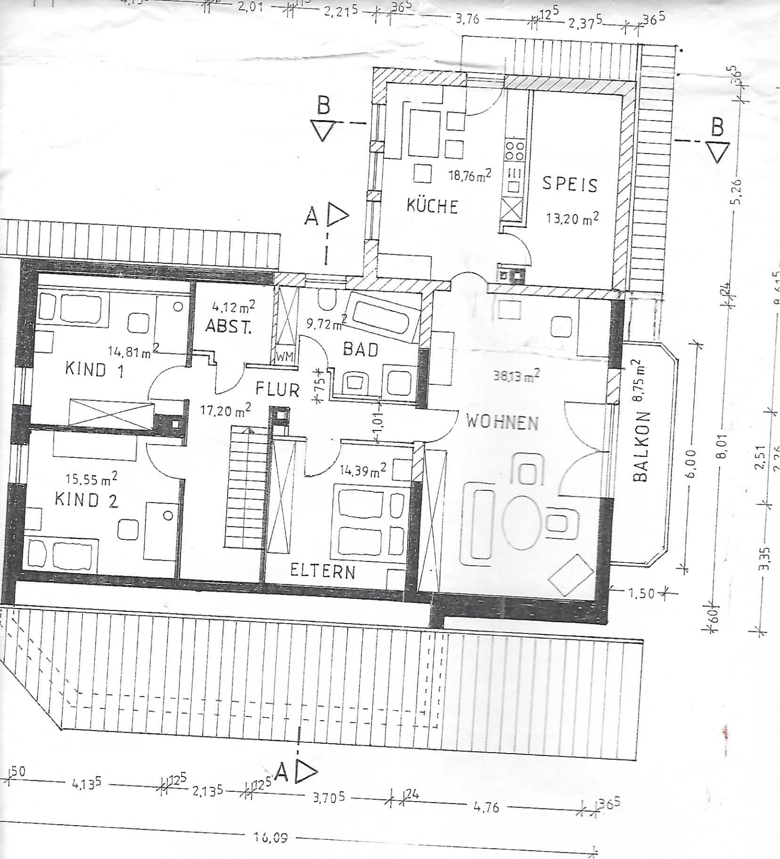
GRUNDRISS-DG
