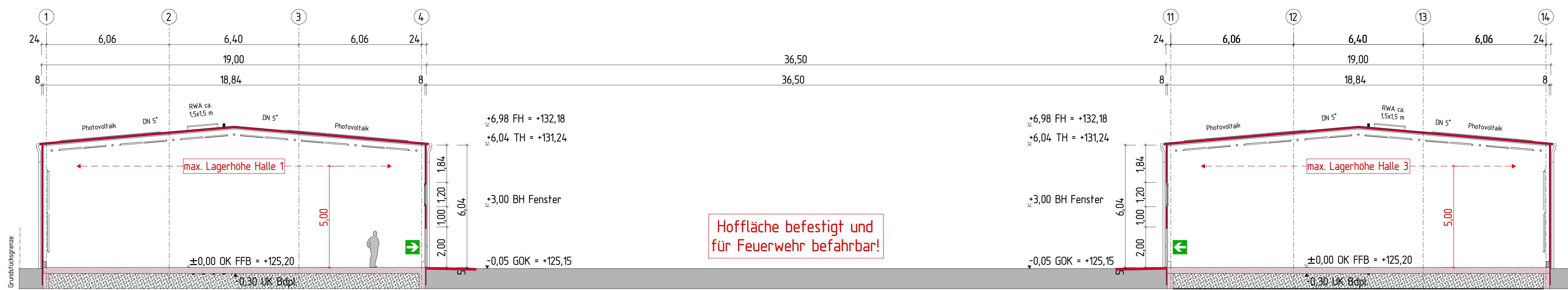
Schnitt A2 - Neubau Halle 1, Bauabschnitt 1
