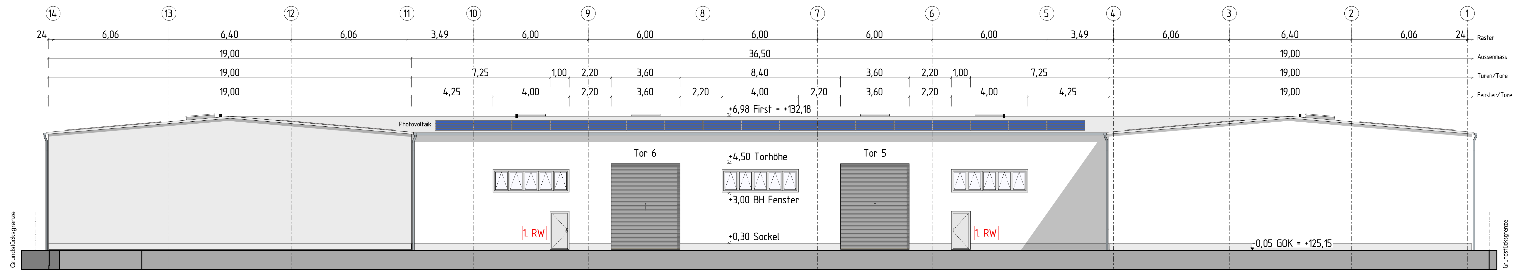
Halle 3, Bauabschnitt 2/3 Ansicht Norden - Neubau Halle 1 bis 3
