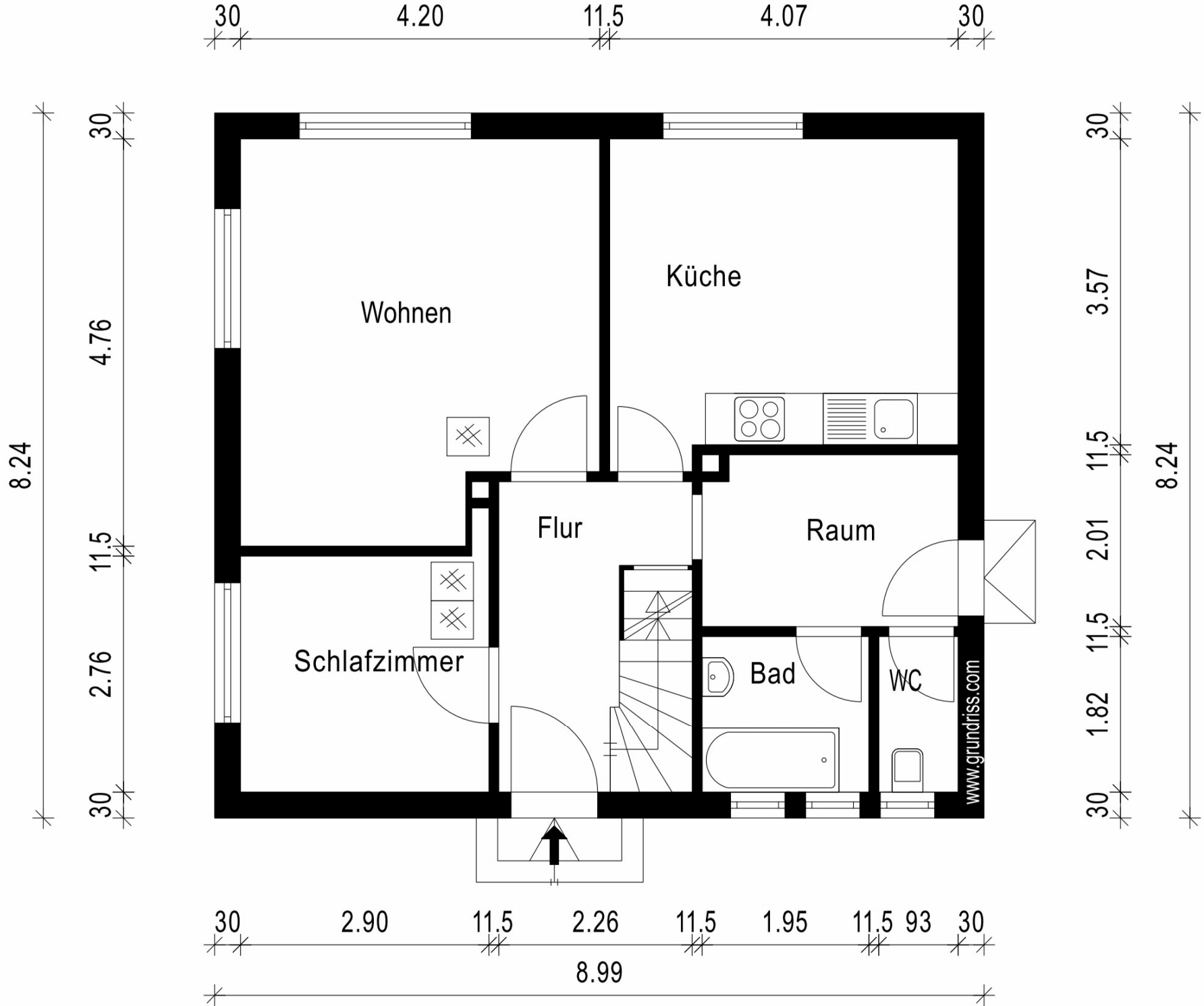
Erdgeschoss
