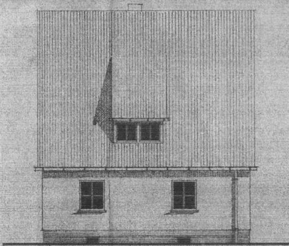
ANSICHT WEST
