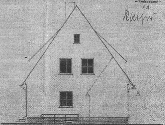
ANSICHT NORD
