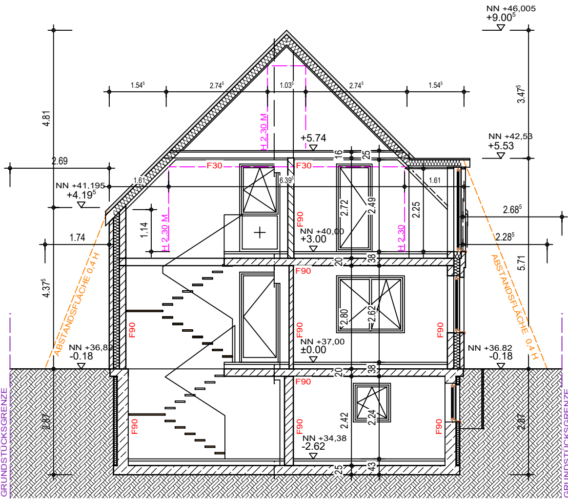
SCHNITT A
