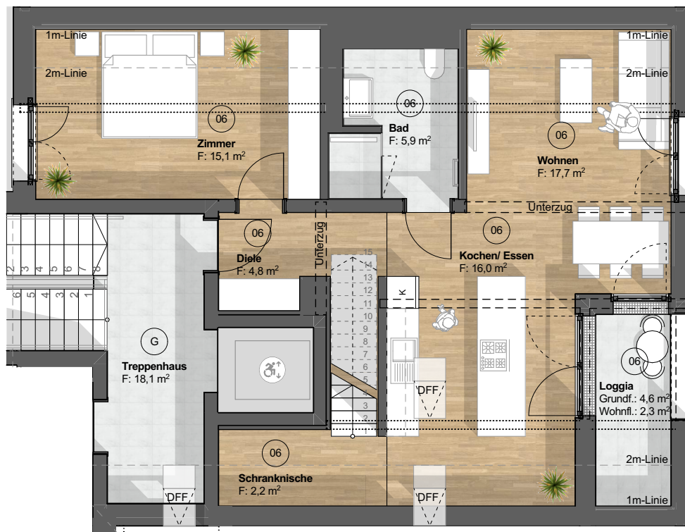
2. Obergeschoss 1:100
