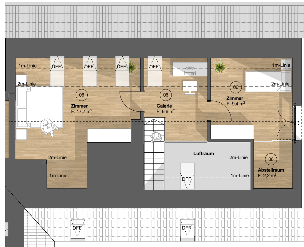
3. Obergeschoss 1:100
