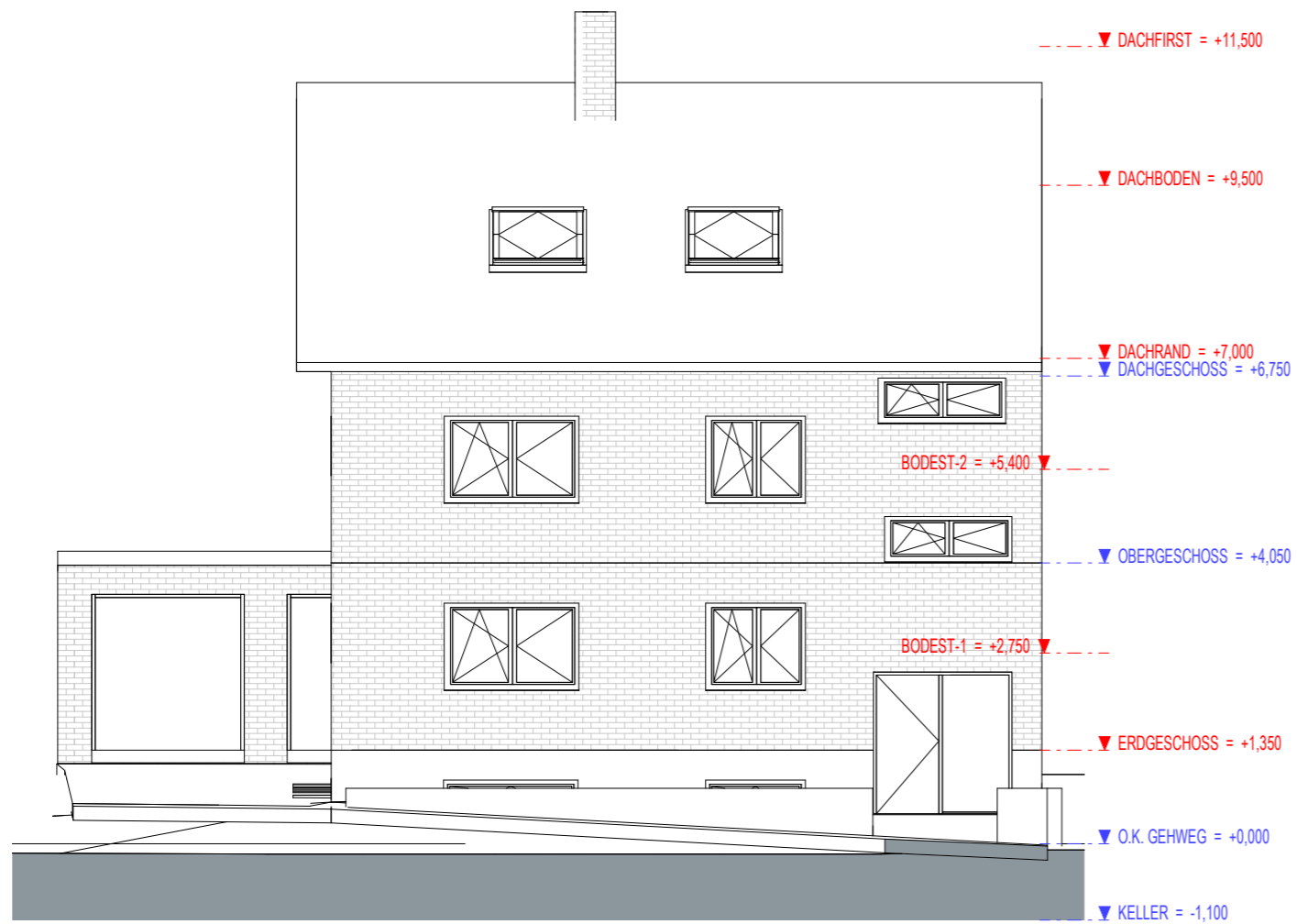
Ansicht 2 - Nord-Ost M 1 : 100
