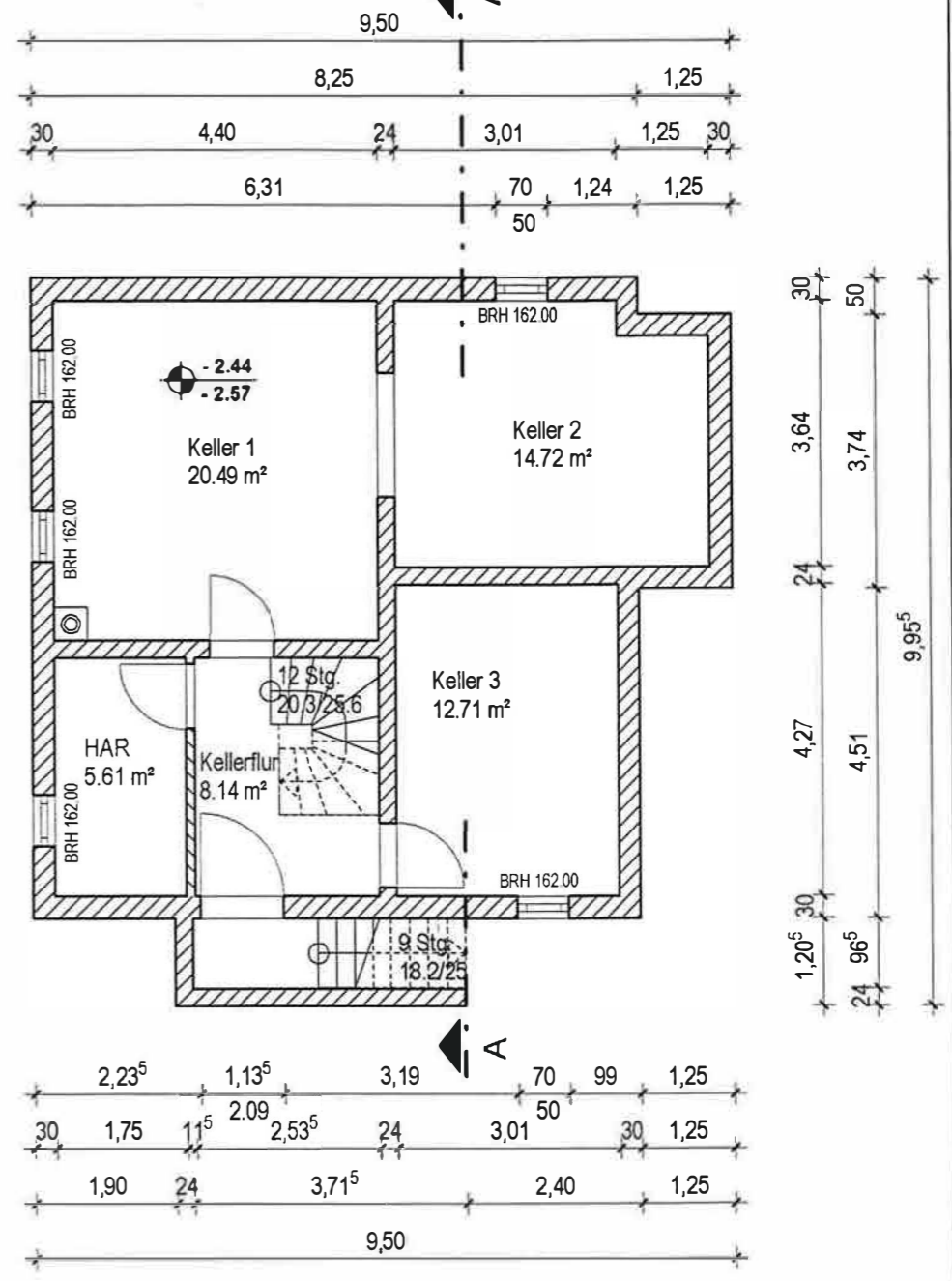
Grundriß Kellergeschoß
