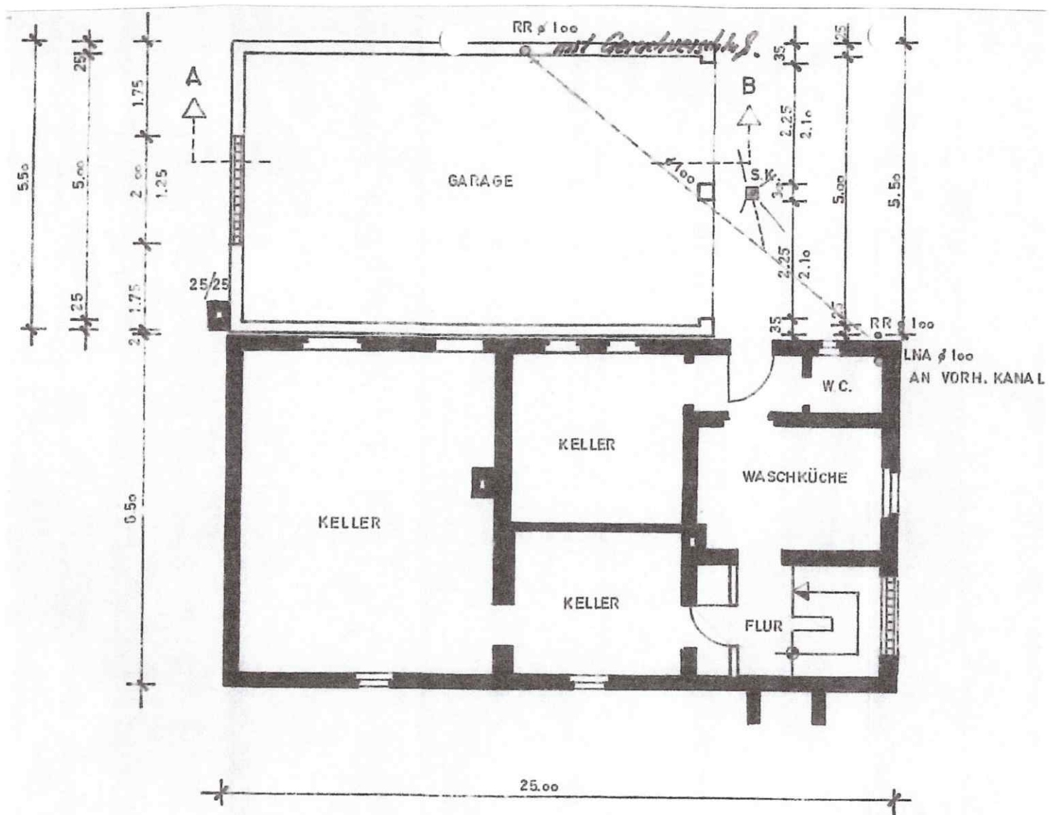
KELLERGESCHOSS
