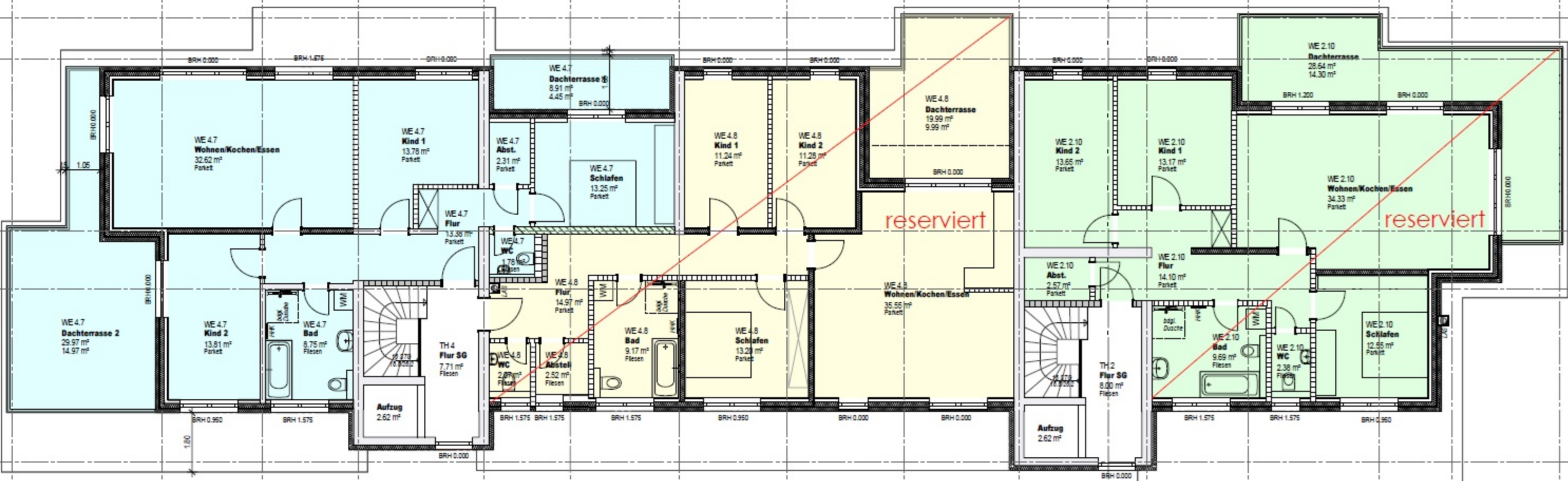
Grundriss Staffelgeschoss Haus 2 und 4
