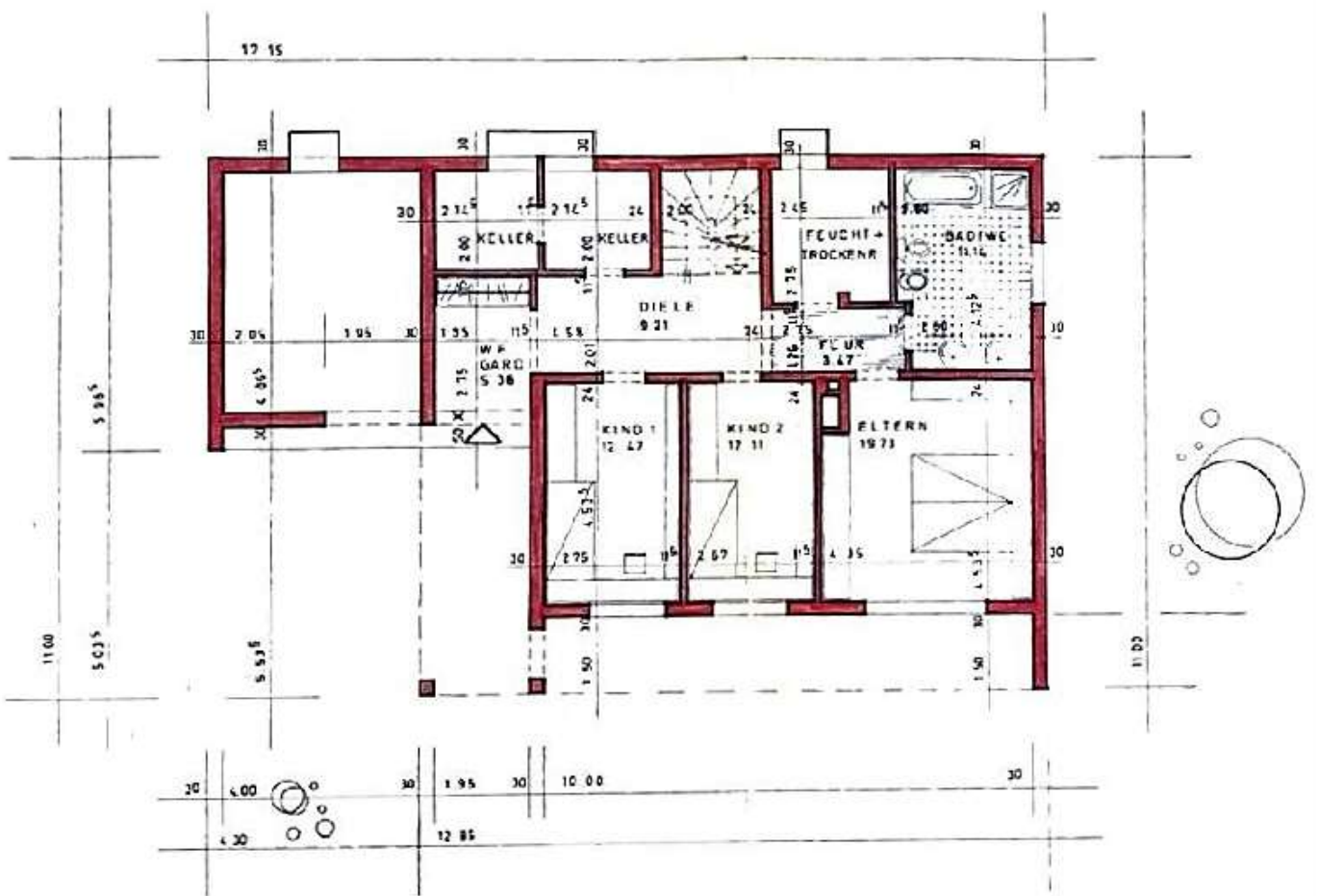
SOCKELGESCHOSS
