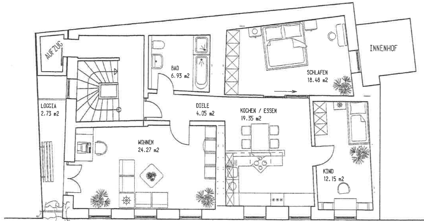
GRUNDRISS 1.OBERGESCHOSS
