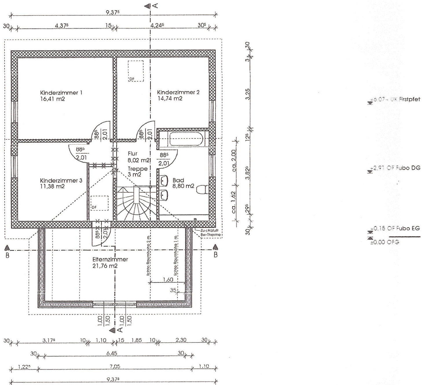
Grundriss Dachgeschoß
