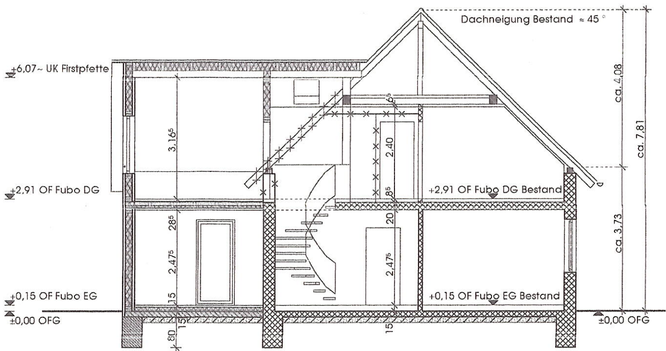
Gebäudeschnitt A
