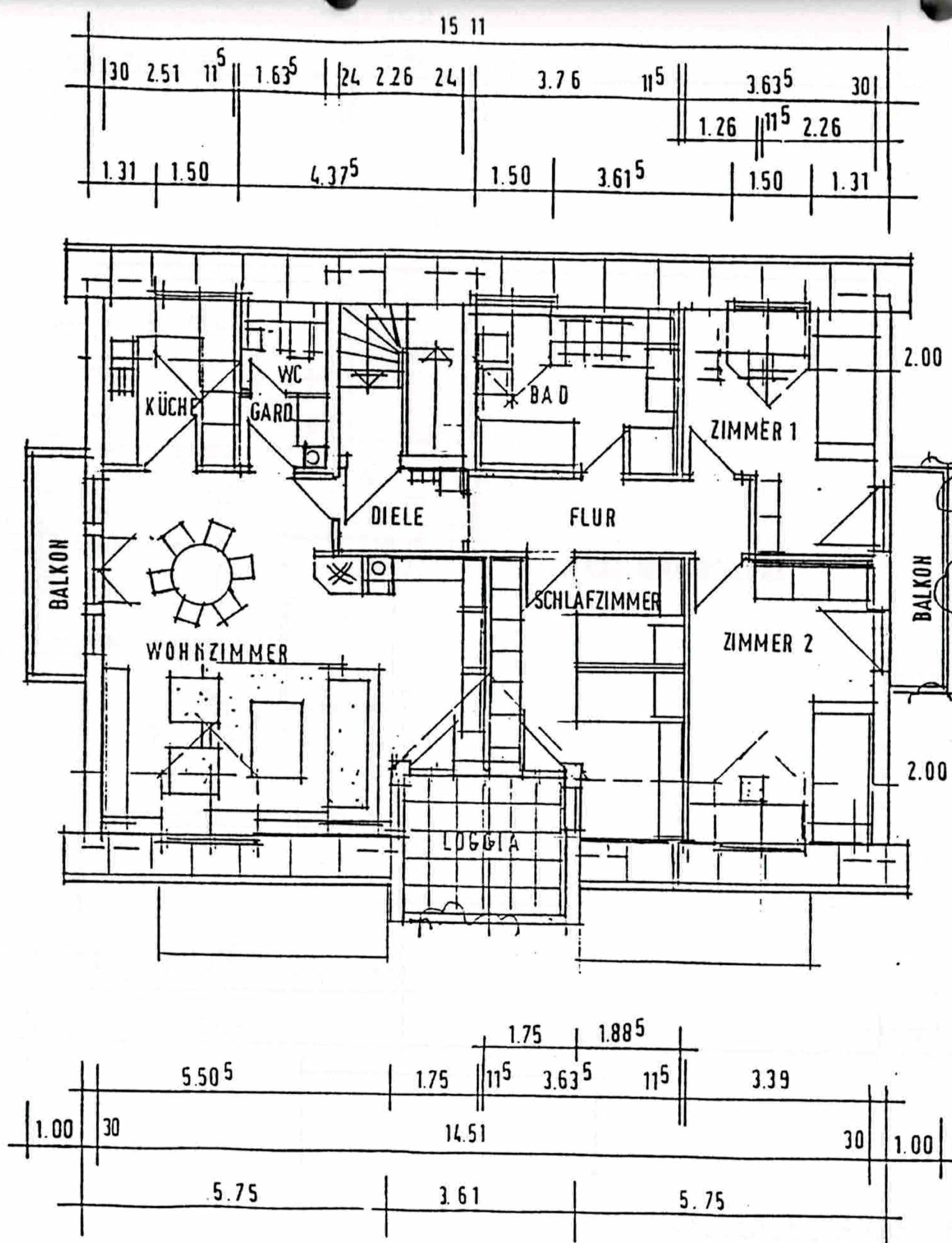
DACHGESCHOSS M 1:100 4-ZI-WOHNUNG NR. 8 118.21 M 2
