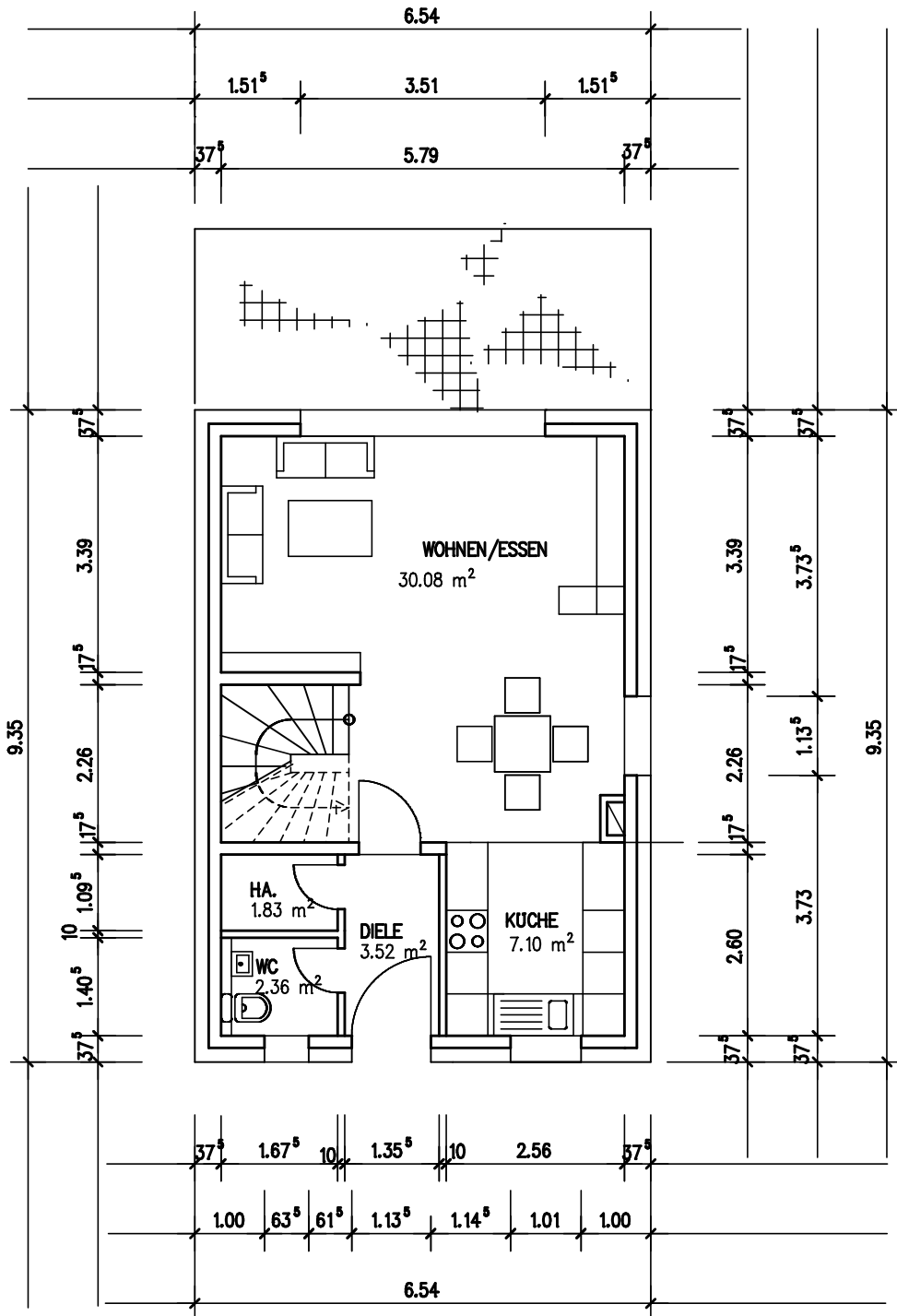
ERDGESCHOSS
