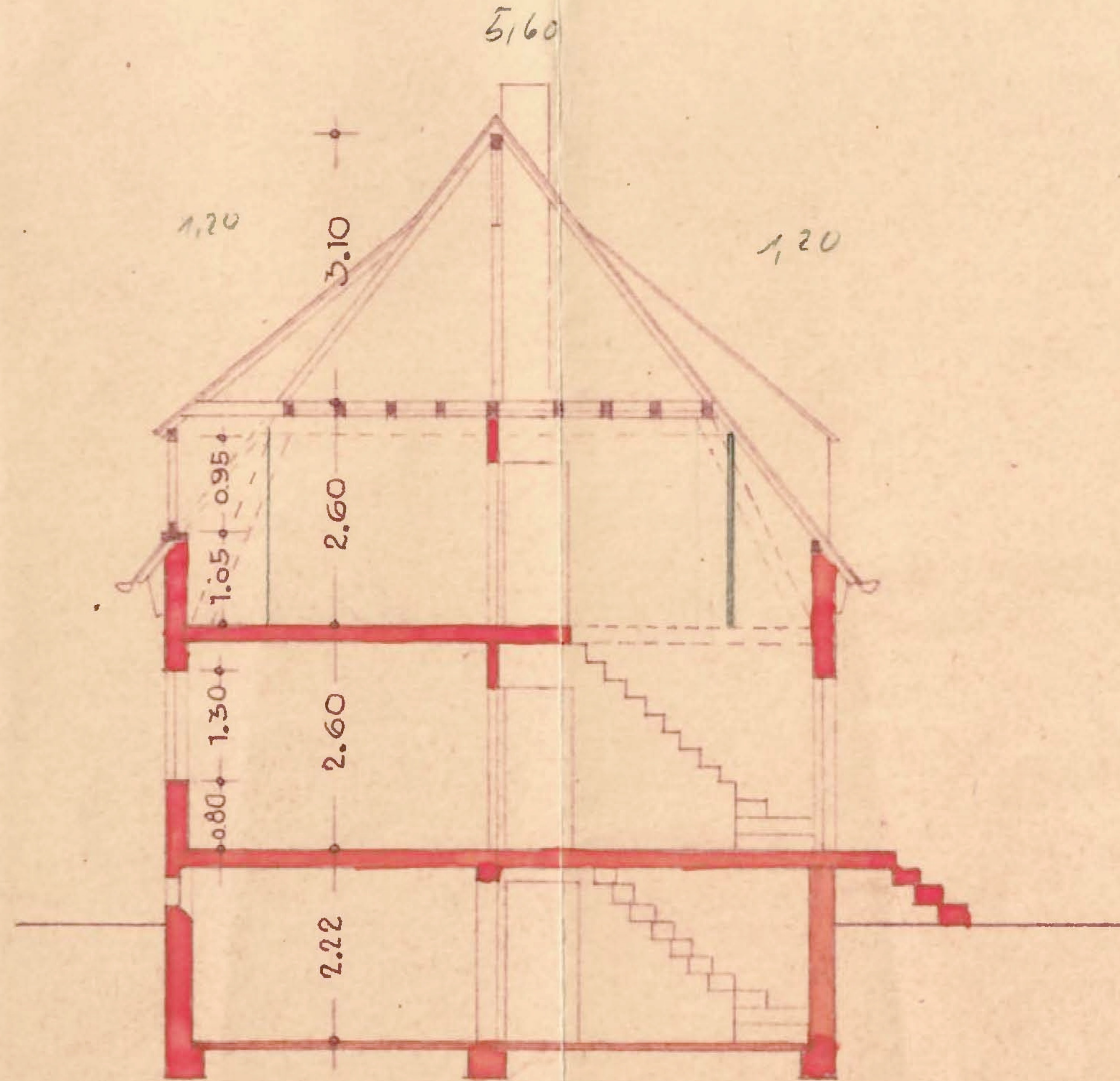
SCHNITT
