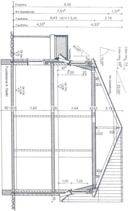
Gebäudeschnitt A - A
