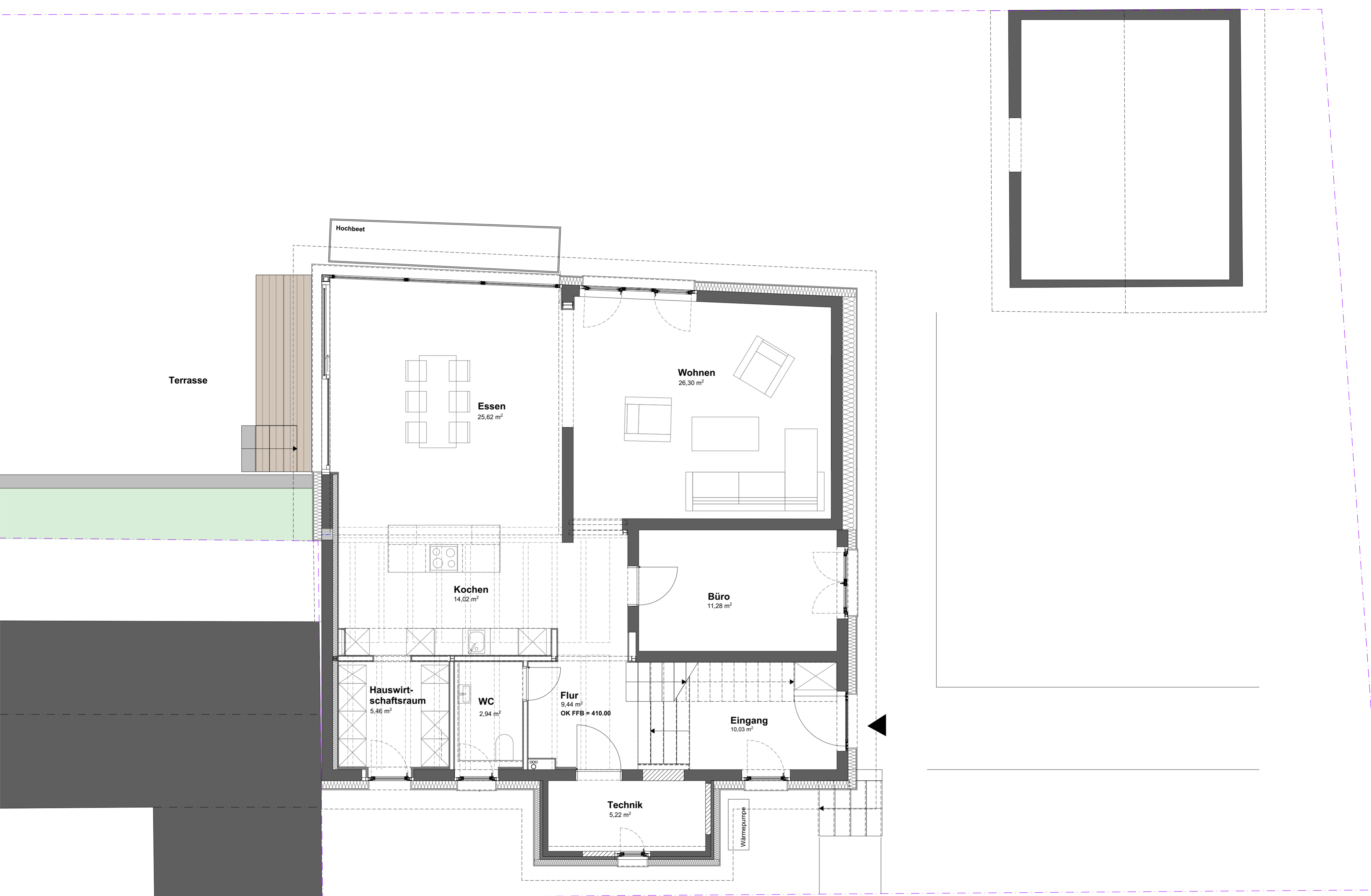
Erdgeschoss
