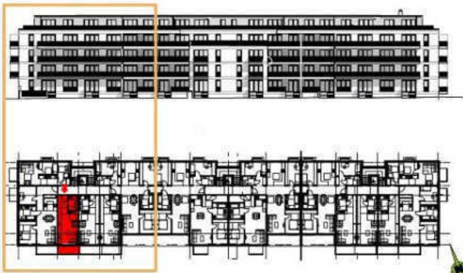
1.OBERGESCHOSS
