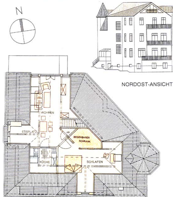
DACHGESCHOSS WOHNUNG 8 ca. 59.50 m 2 +2. OG GESAMTFLÄCHE MAISONNETTEWOHNUNG 80.73 m 2
