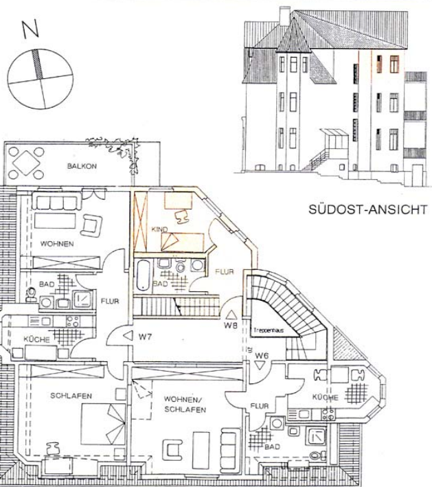
2. OBERGESCHOSS WOHNUNG 8 ca. 21.23 m 2 +DG
