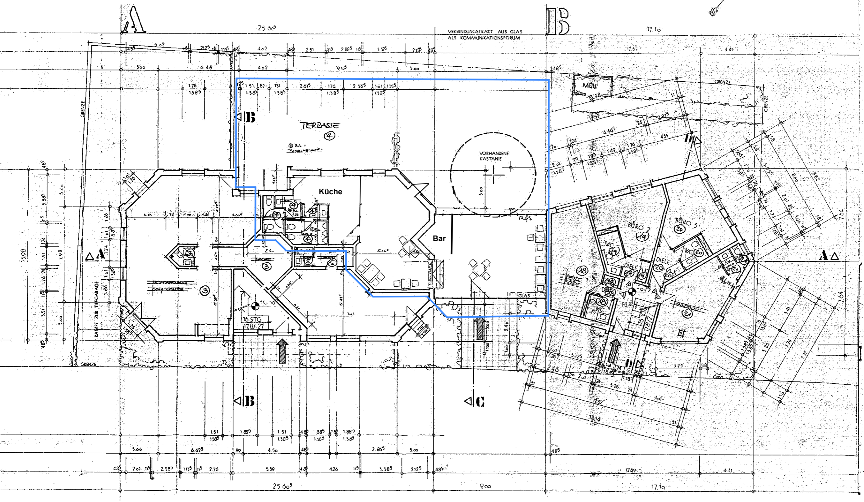
Grundriss Erdgeschoss
