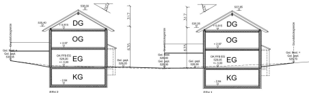
Schnitt A-A M = 1/200
