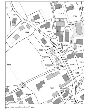
Lageplan M = 1/1000 Gemarkung : Mittbach Flur Nr.: Teilstück von 1698
