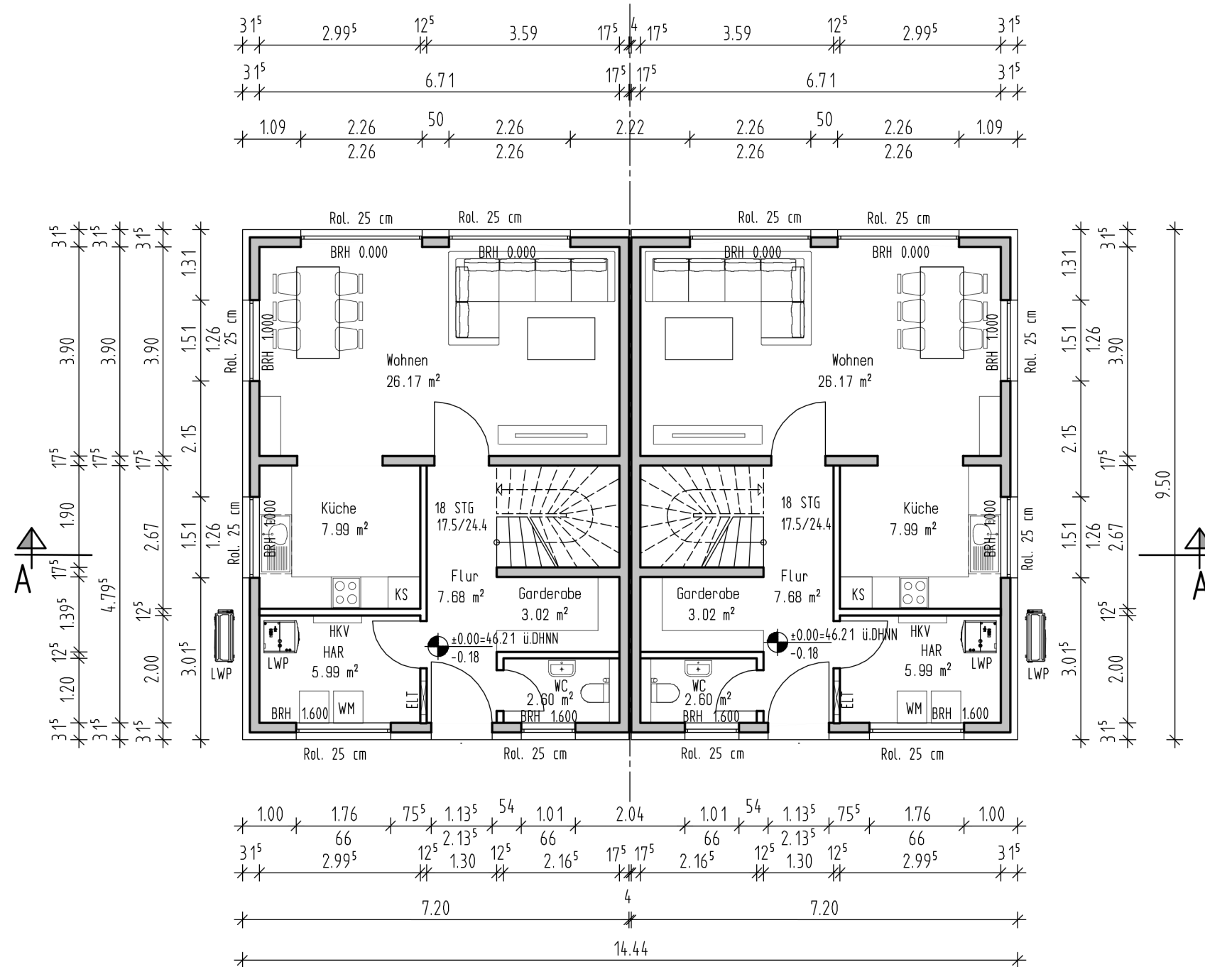
ERDGESCHOSS
