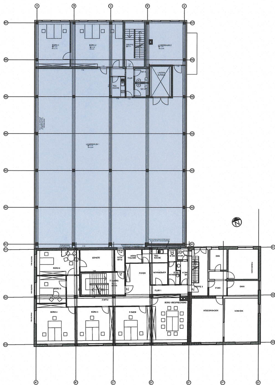
Grundriss 1.OG Zementierhaus Peißenberg
