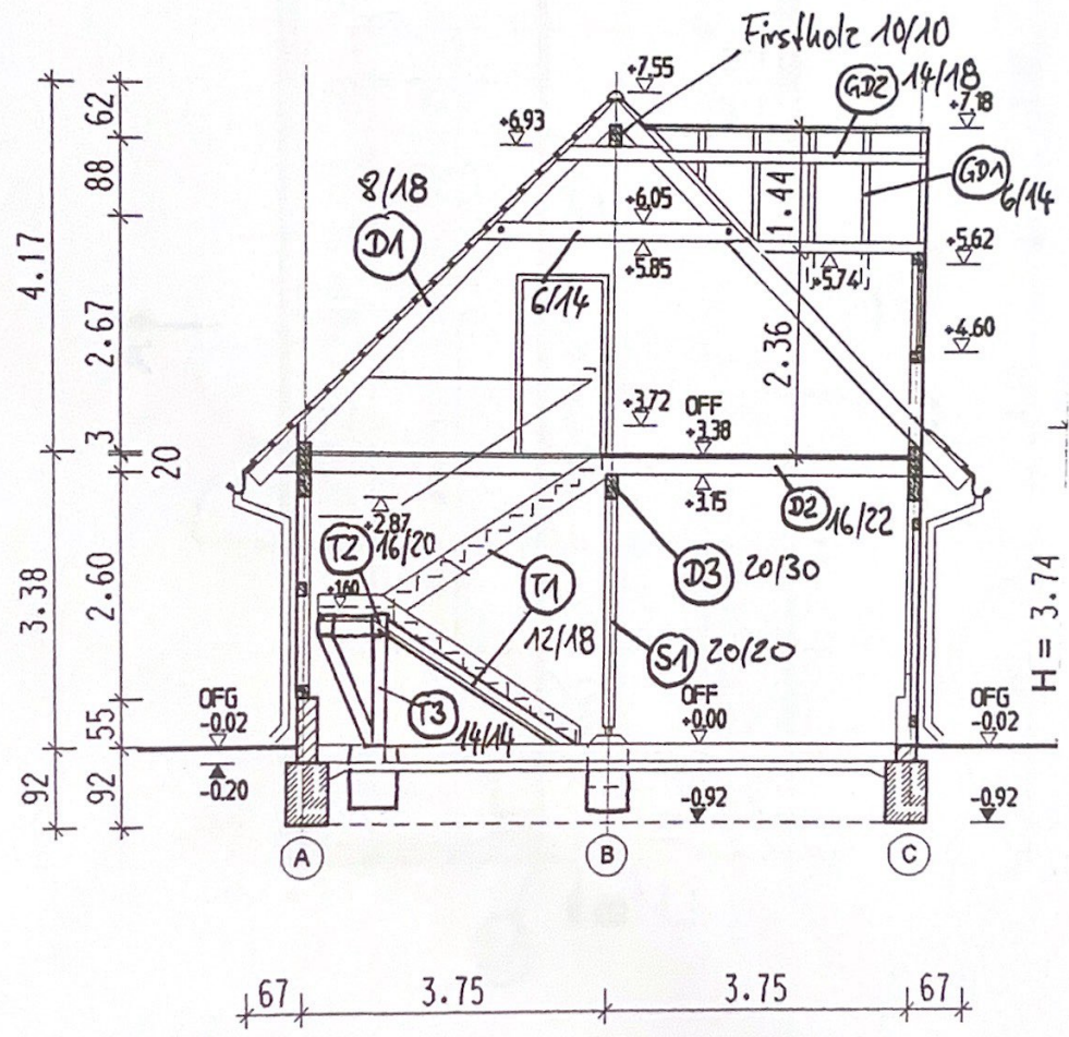
Schnitt A-A
