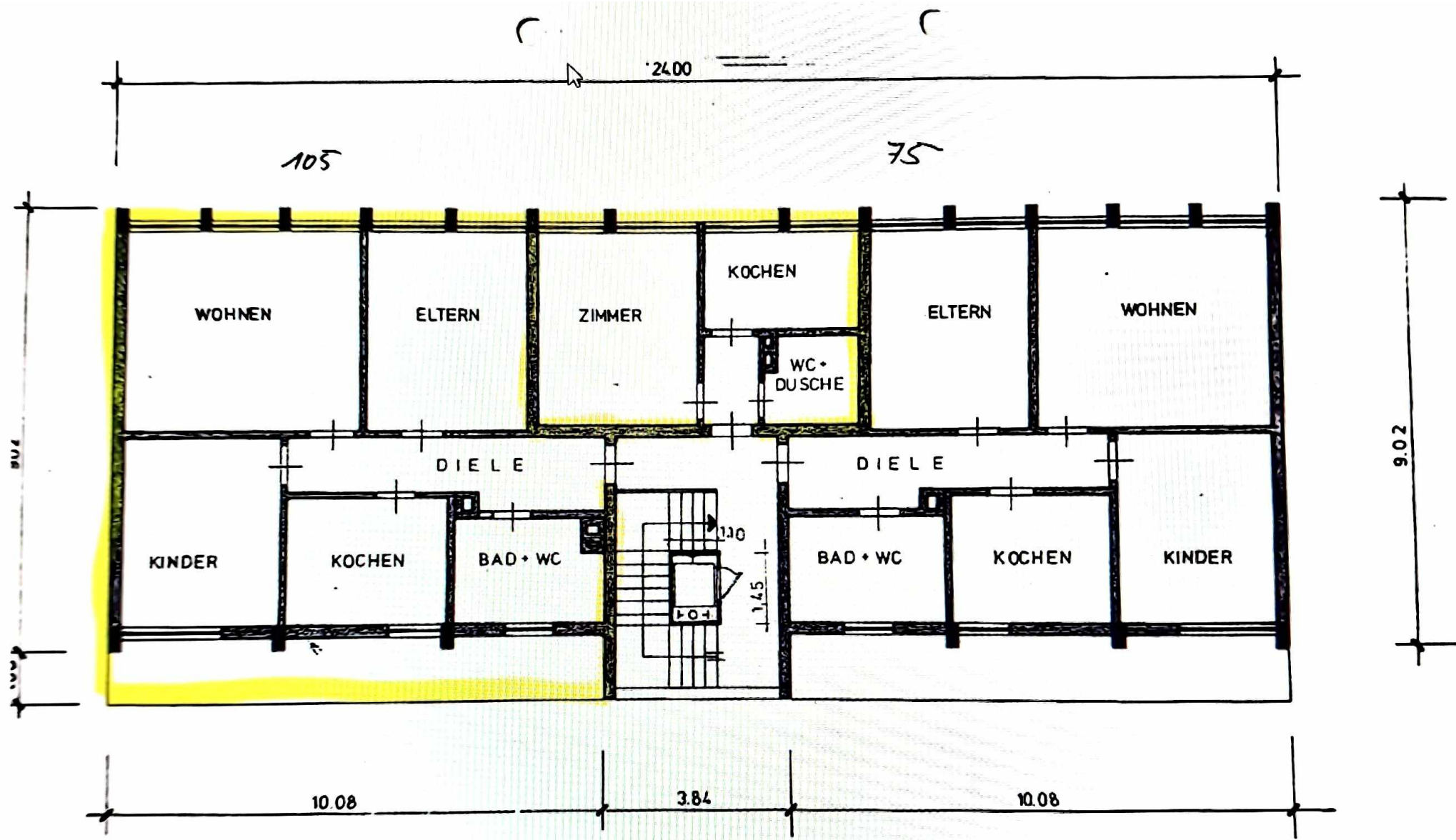
1. + 2. OBERGESCHOSS (BESTEHEND)
