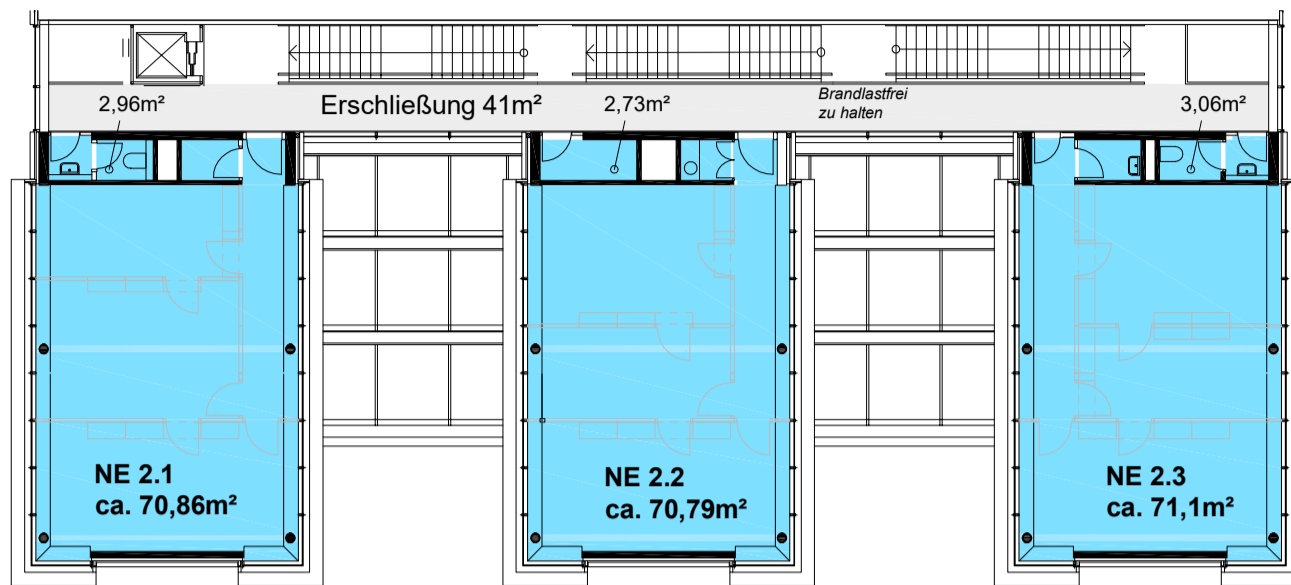
2. Obergeschoss
