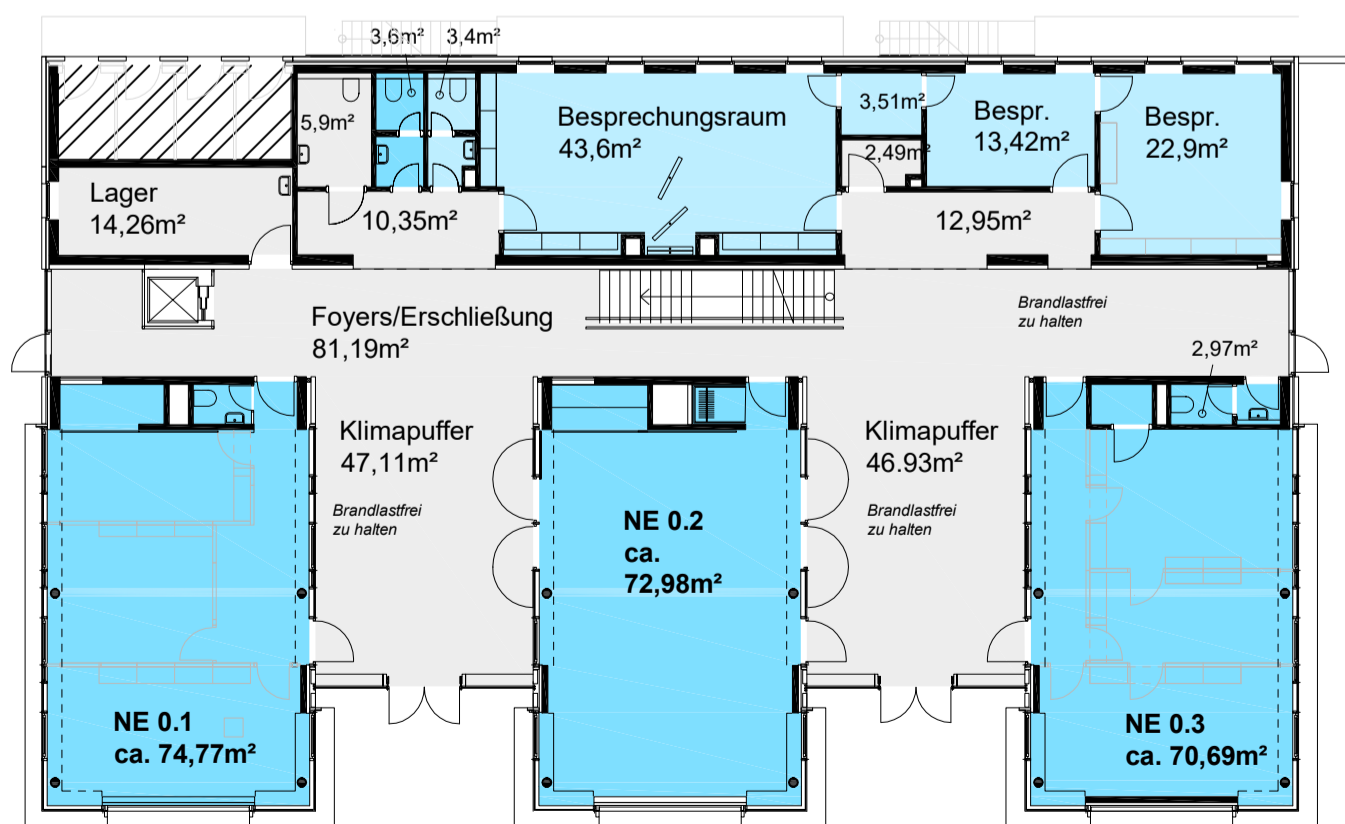
Erdgeschoss
