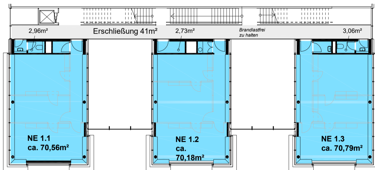
1. Obergeschoss
