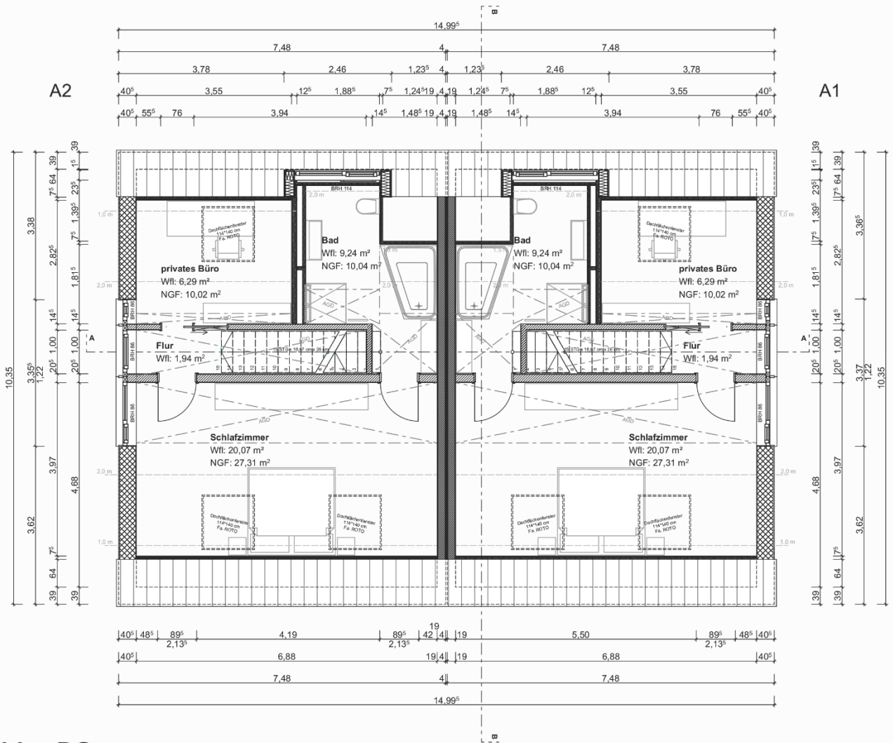
Grundriss DG
