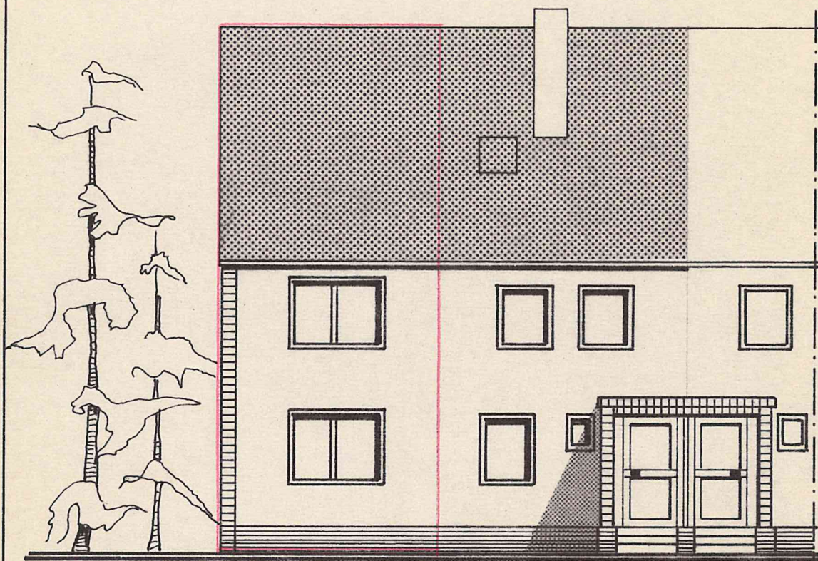
WESTANSICHT
