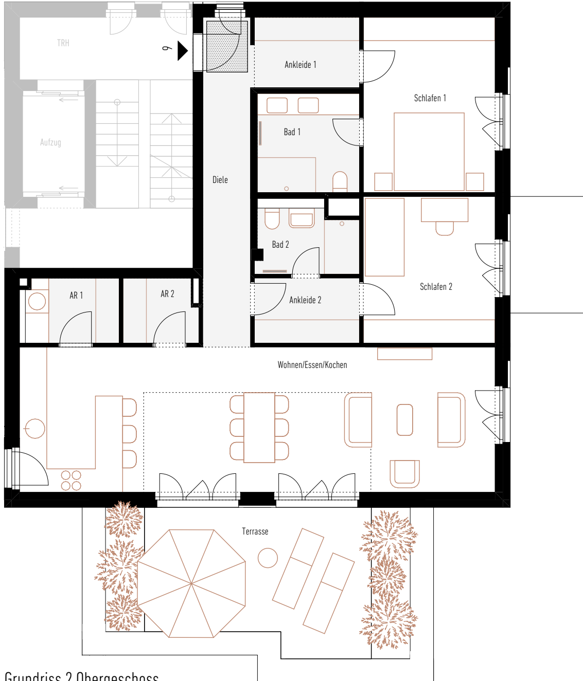
Grundriss 2.Obergeschoss
