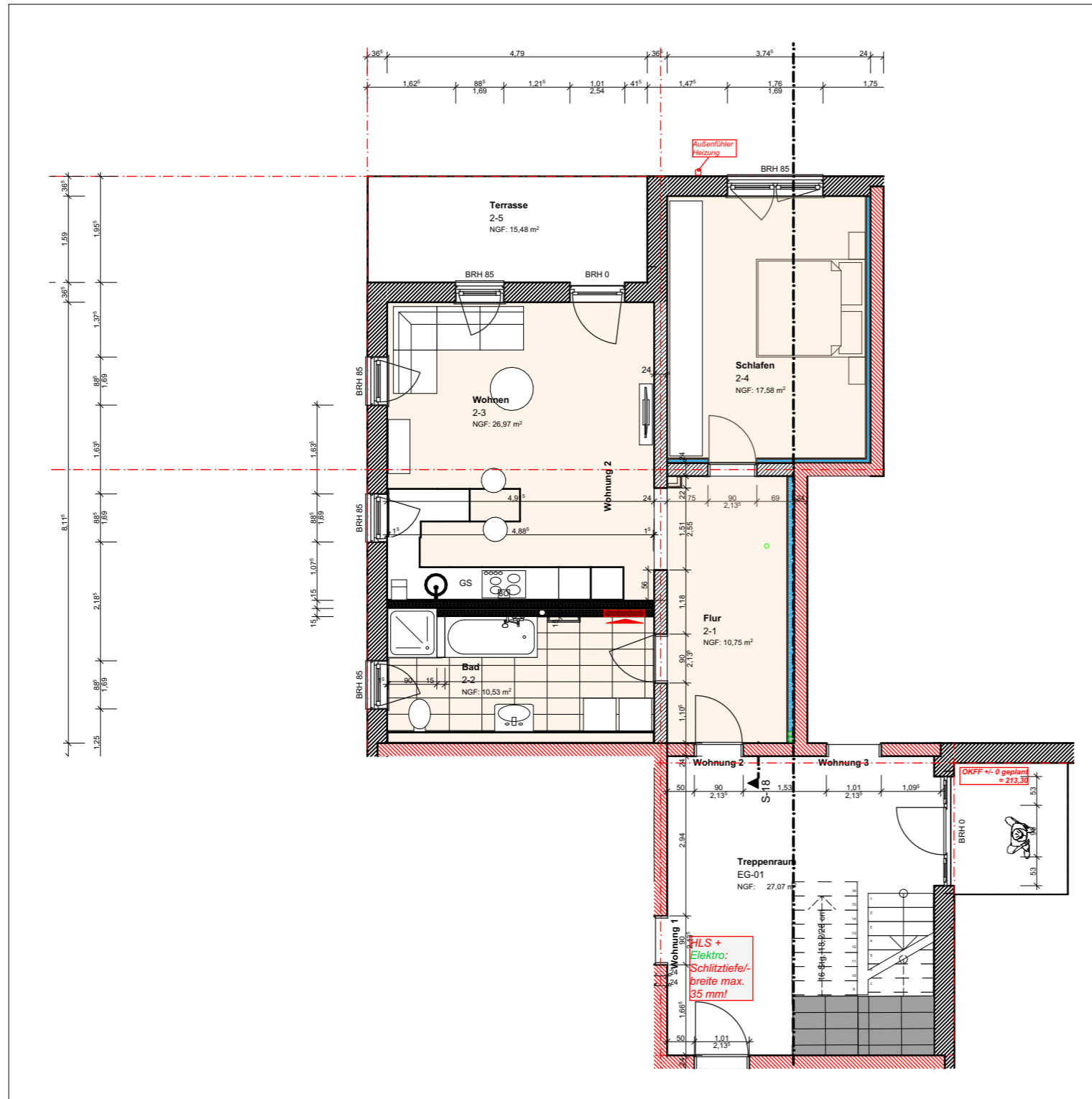
Wohnungsgrundriss (Darstellung mit Treppenhaus) nach Planungsstand mit Einrichtungsvorschlag
